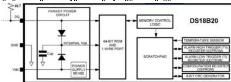
ნახაზი №2 – DS18B20-ის ბლოკ-სქემა
