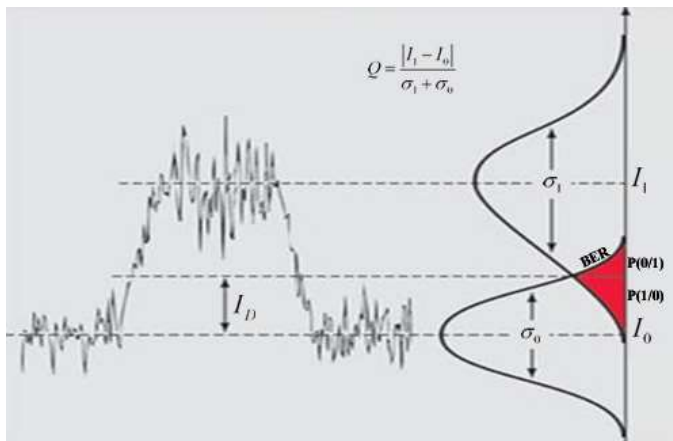
ნახ. 1. თანაფარდობა „0“ და „1“ დონეების 2. BER = \Psi(Q) დამოკიდებულების
