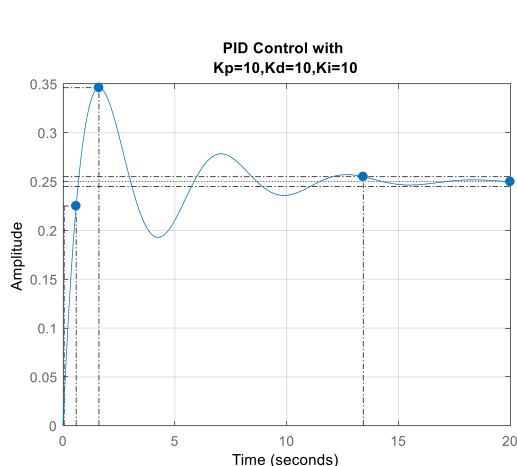
ა) K_p=10, K_d=10, K_i=10
