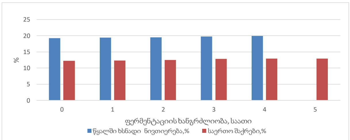
დიაგრამა 5. მიღებულ წვენში წყალში ხსნადი ნივთიერებებისა და საერთო შაქრების რაოდენობის ცვლილება 0,1% პექტოლიტური ფერმენტული პრეპარატის დამატებისას წყავის დურდოში 40-50°C-ზე
