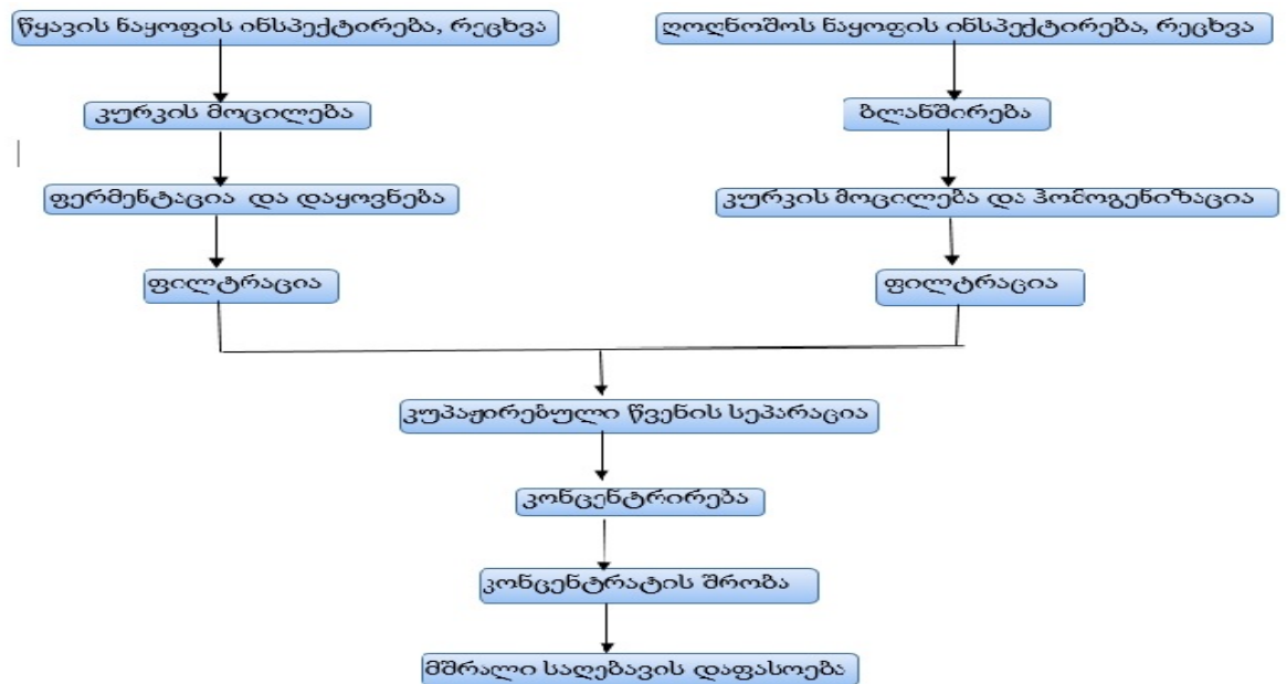
ნახაზი 4. ბუნებრივი საკვები საღებარის წარმოების ტექნოლოგიური სქემა წყავისა და ღოღნოშოს კუპაჟირებული წვენისაგან.
