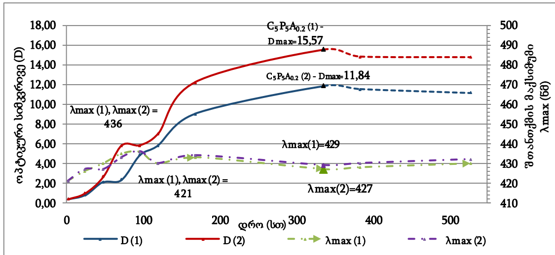
ნახ. 12. ვერცხლის ნანოკომპოზიტების P_5C_5A_{0.2} -ის ოპტიკური სიმკვრივის (D) და შთანთქმის მაქსიმუმის ( \lambda_{max} , ნმ) ცვლილება დროში. წარმოდგენილია ორი პარალელური ცდის შედეგი
