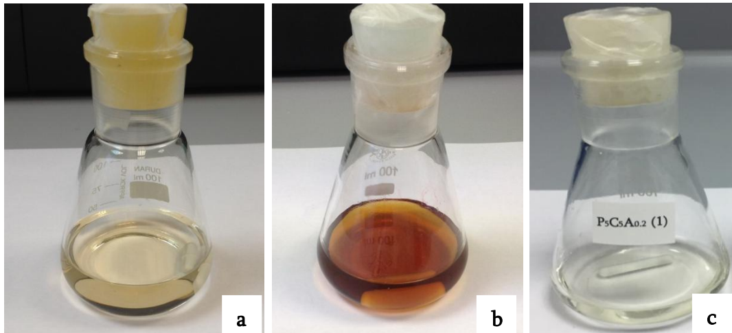
ნახ. 1. ვერცხლის ნანოკომპოზიტ P_{10}A_1 -ის საკვლევი ხსნარი ეთანოლში დასხივებამდე (a), დასხივებიდან 24 სთ-ის შემდეგ (b) და მასტაბილიზირბელი დანამატის გარეშე (c)
