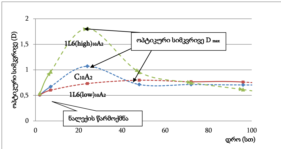
ნახ. 9. ვერცხლის ნანოკომპოზიტების C_{10}A_2 , 1L6(low)_{10}A_2 და 1L6(high)_{10}A_2 -ის ოპტიკური სიმკვრივის დროსთან დამოკიდებულება
