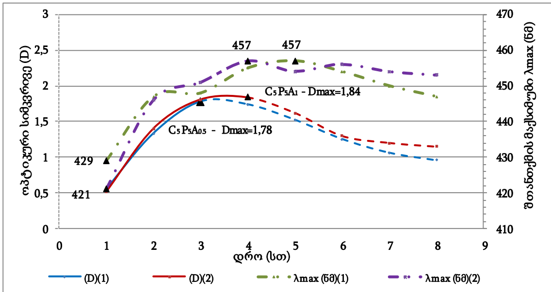
ნახ. 11. ვერცხლის ნანოკომპოზიტების P_5C_5A_1 -ის და P_5C_5A_{0.5} -ის ოპტიკური სიმკვრივის (D) და შთანთქმის მაქსიმუმის ( \lambda_{max} , ნმ) ცვლილება დროში
