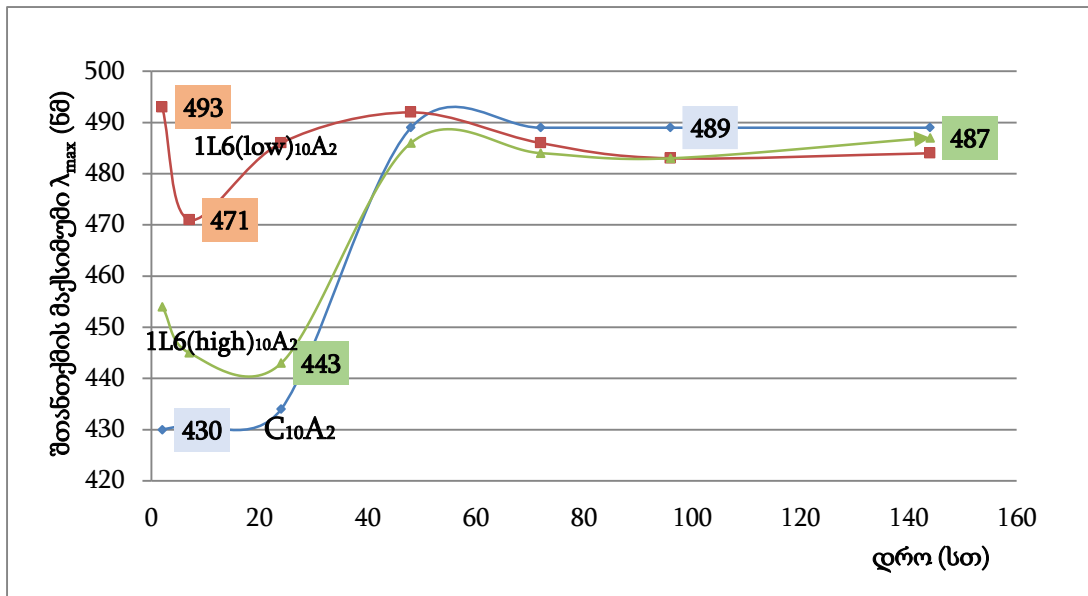
ნახ. 10. ვერცხლის ნანოკომპოზიტების C_{10A2} , 1L6(low)_{10A2} და 1L6(high)_{10A2} -ის შთანთქმის მაქსიმუმის ( \lambda_{max} ნმ) ცვლილება დროში
