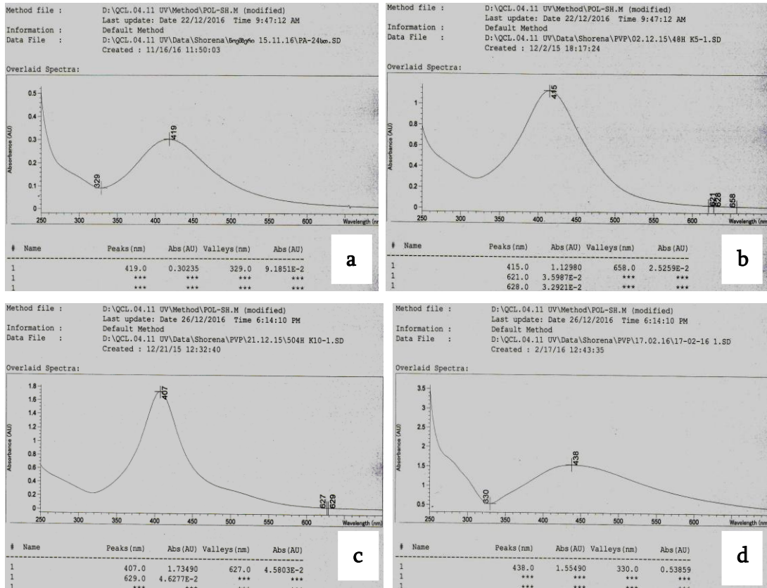
ნახ. 2. ვერცხლის ნანოკომპოზიტ P10A1-ის უი-სპექტრი სინათლეზე დაყოვნებიდან 24,0 სთ-ის (a), 48,0 სთ-ის შემდეგ (b), 500,0 სთ-ის (c) და 2000,0 სთ-ის შემდეგ (d)
