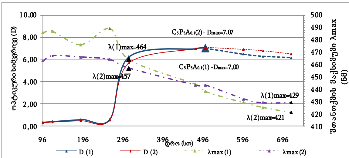
ნახ. 13. ვერცხლის ნანოკომპოზიტების P_5C_5A_{0.1} -ის ოპტიკური სიმკვრივის (D) და შთანთქმის მაქსიმუმის ( \lambda_{max} , ნმ) ცვლილება დროში. წარმოდგენილია ორი პარალელური ცდის შედეგი
