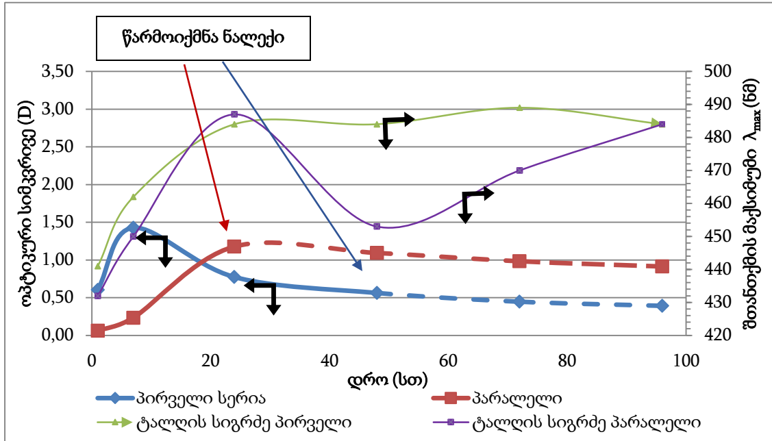
ნახ. 7. ვერცხლის ნანოკომპოზიტ 1L6(high) 10 A 1 -ის ოპტიკური სიმკვრივის (D) და შთანთქმის მაქსიმუმის ( \lambda_{max} , ნმ) ცვლილება დროში
