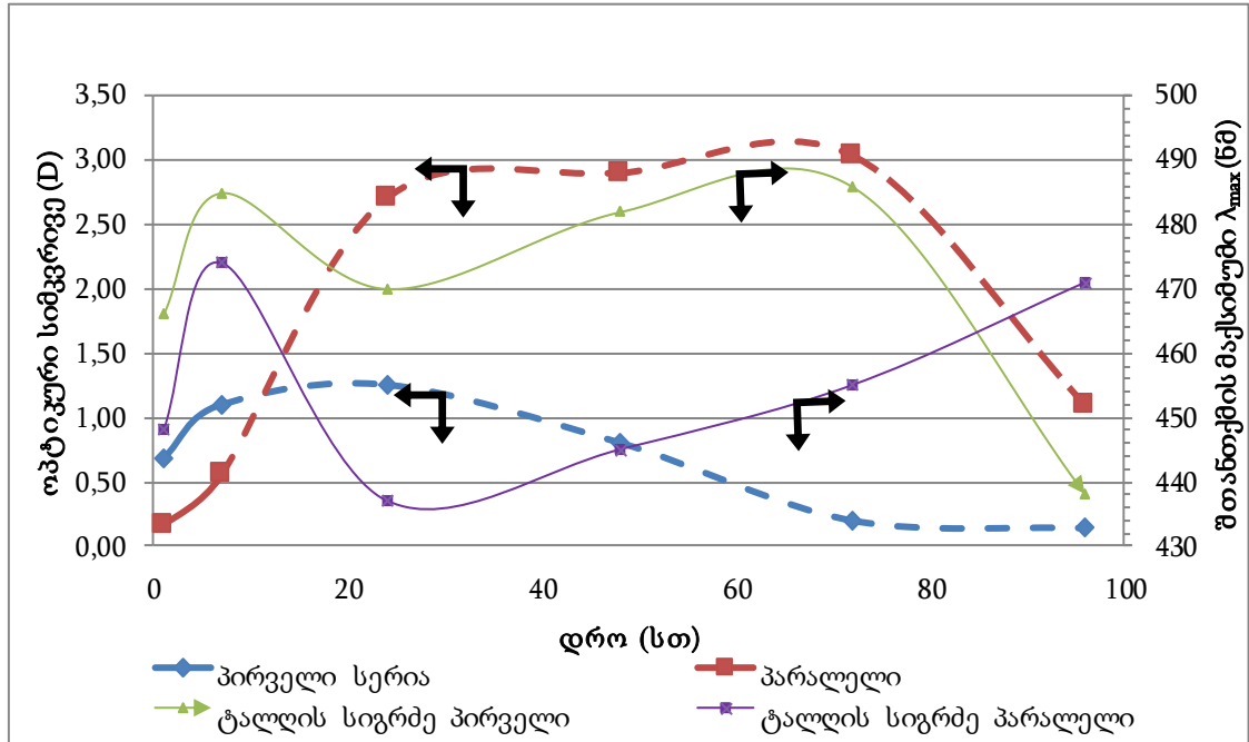
ნახ. 6. ვერცხლის ნანოკომპოზიტ 1L6(low) 10 A 1 -ის ოპტიკური სიმკვრივის (D) და შთანთქმის მაქსიმუმის (λ max , ნმ) ცვლილება დროში
