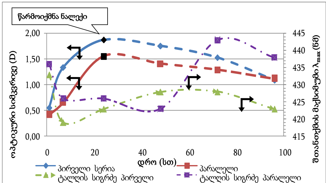
ნახ. 5. ვერცხლის ნანოკომპოზიტ C_{10}A_1 -ის ოპტიკური სიმკვრივის (D) და შთანთქმის მაქსიმუმის ( \lambda_{max} , ნმ) ცვლილება დროში
