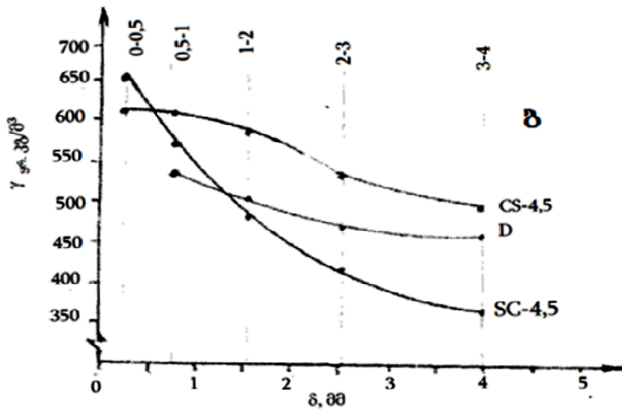
ნახ.4 . ყვარლის ფიქლის 2(ა) ან 5%-იანი (ბ) ნახშირის დამატებით შედგენილი ნარეგების აფუებით მიღებული მასალების მოცულობითი სიმკვრივე.
