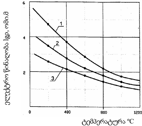
ნახ. 8. სხვადასხვა ფრაქციის კოქსწვრილას ელექტროწინალობის ცვლილება 0-1200°C ტემპერატურულ ინტერვალში: 1- 0-5მმ; 2 - 5-20მმ; 3 - 20-25მმ.
