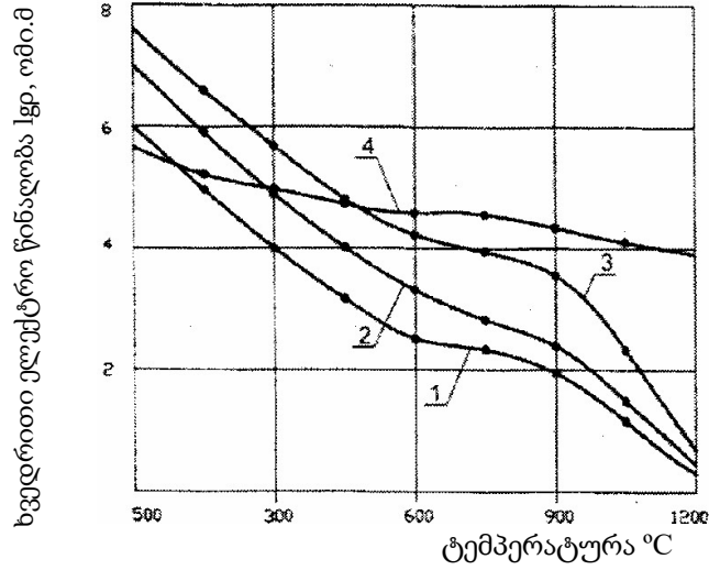
ნახ. 5. სხვადასხვა ხარისხის მადნების ელექტროწინაღობის დამოკიდებულება ტემპერატურაზე: 1 – Mn -49%; 2. – Mn -44%; 3. – Mn -35%; 4. – კვარციტი.
