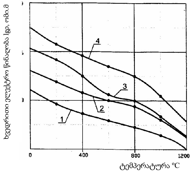
ნახ. 6. სხვადასხვა შედგენილობის კაზმების ელექტროწინაღობის დამოკიდებულება ტემპერატურაზე: 1. მადანი +100% კოქსი; 2. მადანი +70% კოქსი +30% ნახშირი; 3. მადანი+100% ნახშირი; 4. მადანი + 100% ნახშირი + კვარციტი
