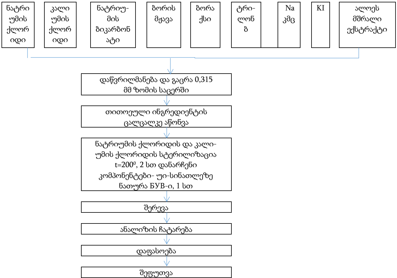
სქემა 4. კბილის მშრალი ელექსირის მიღების ტექნოლოგია
