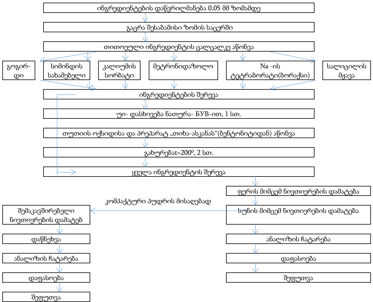
სქემა 1. სამკურნალო-პროფილაქტიკური პუდრის მიღების ტექნოლოგია
