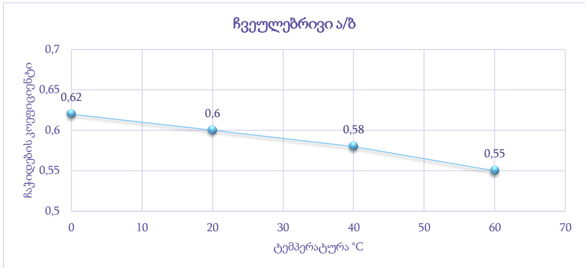
ნახ. 51. ჩაჭიდების შედეგები ტემპერატურულ დიაპაზონში ა/ზ-ის საფარისათვის
