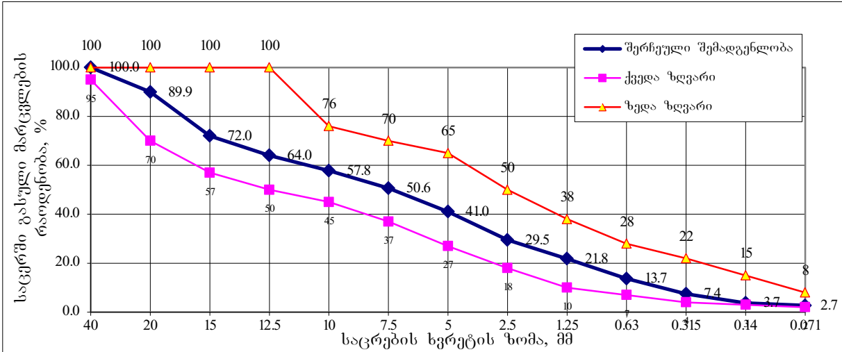
ნახ. 9. ცხელი, წვრილმარცვლოვანი, მკვრივი „ბ“ ტიპის II მარკის ასფალტბეტონის ნარევისათვის მინერალური ნაწილის გრანულომეტრიული (მარცვლოვანი) შემადგენლობა
