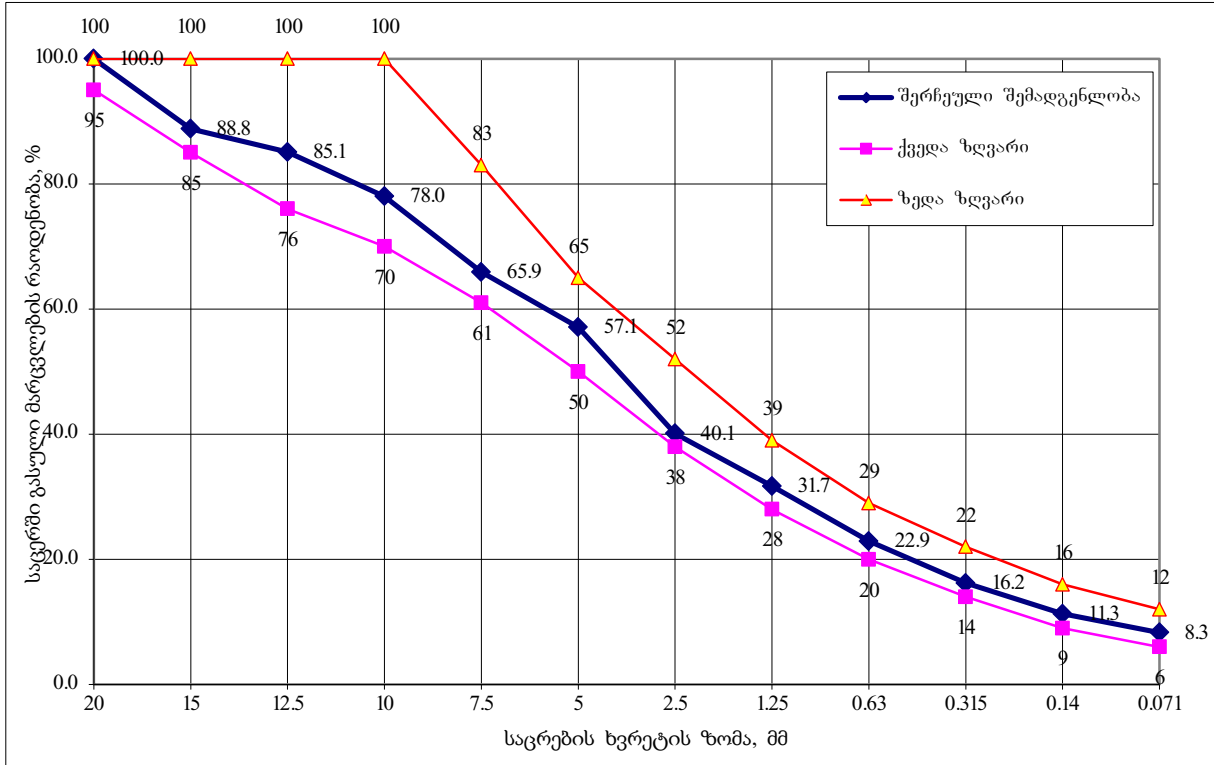
ნახ. 10. ცხელი, წვრილმარცვლოვანი, მკვრივი „ბ“ ტიპის II მარკის ასფალტბეტონის ნარევისათვის მინერალური ნაწილის გრანულომეტრიული (მარცვლოვანი) შემადგენლობა
