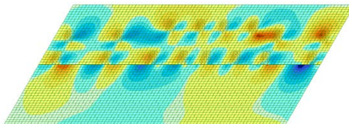
ნახ. 35. მგრები მომენტის იზოვლები
