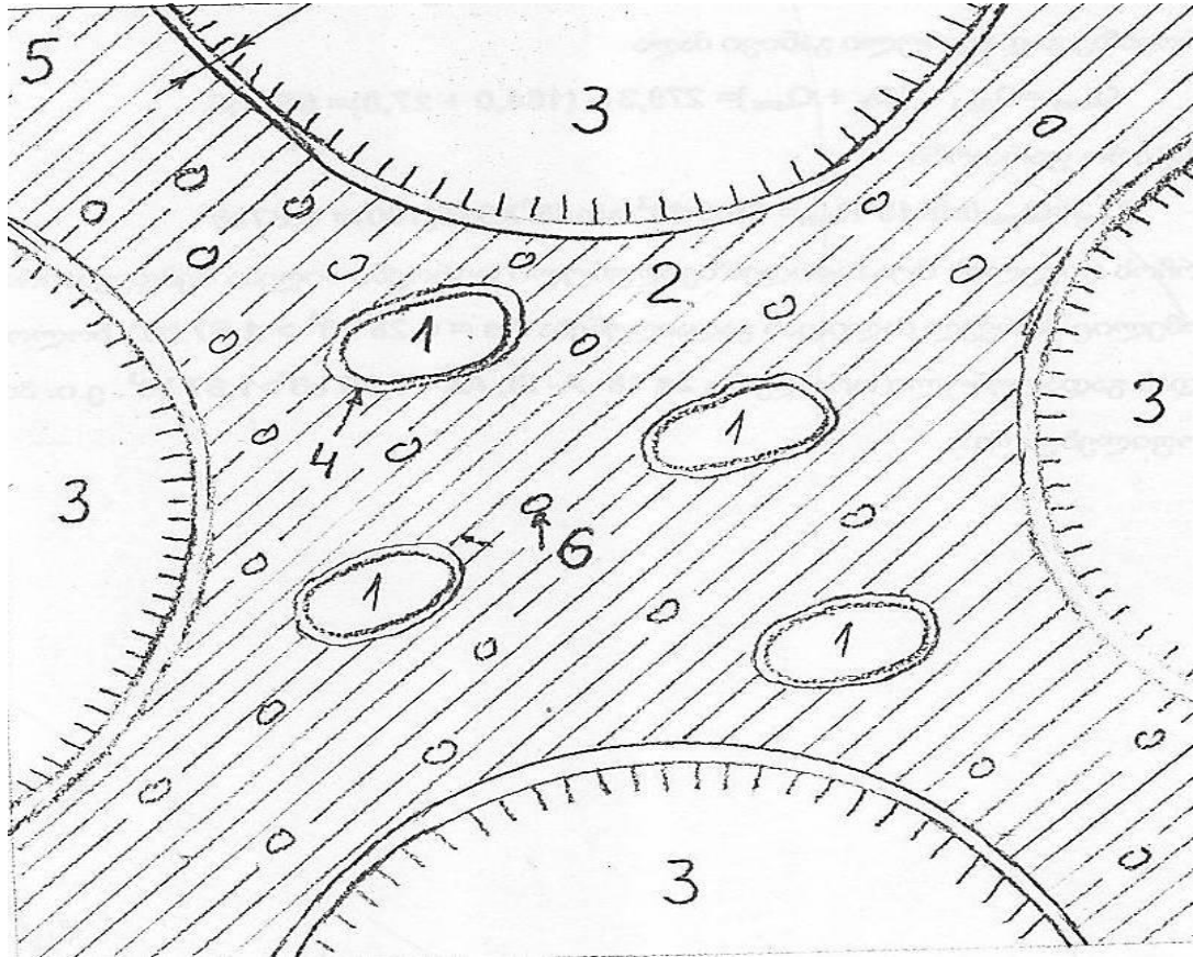
ნახ. 1.4 3 დღე-ღამის ასაკში გამყარებული ბეტონის სტრუქტურული სქემა
