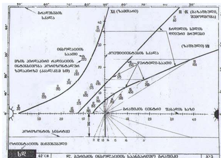
სურ. 9. ლ. ბერიძის ინსოლაციის საანგარიშო გრაფიკი
