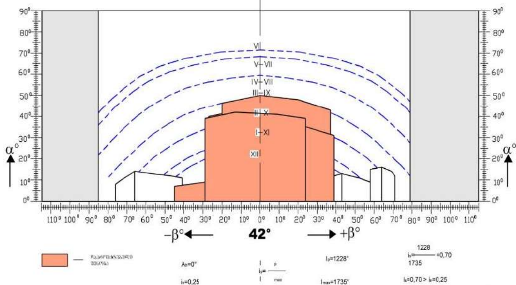
ი ს ო ლ ა ც ი ი ს გ ა ა ნ გ ა რ ი შ ე ბ ა (ვიზუალურ - სივრცითი მეთოდი) სერი ფანტომაგ - ფ-1
