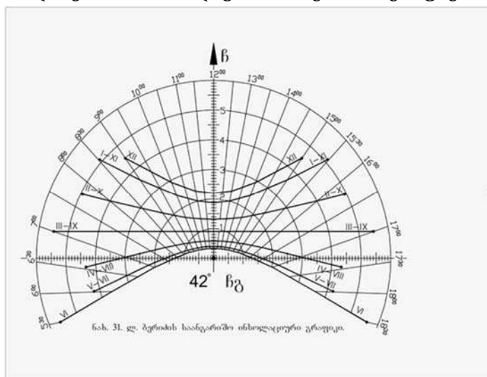
სურ. 10. ლ. ბერიძის ინსოლაციის საანგარიშო გრაფიკი
