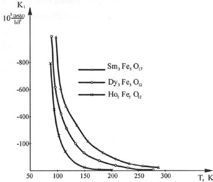
ნახ. 2 K_1 კონსტანტას დამოკიდებულება ტემპერატურაზე სხვადასხვა ფერიტ-მოწზე
