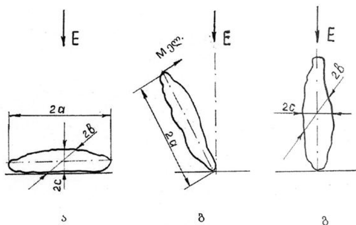
ნახ. 1. ელექტროდზე მდებარე ნაწილაკის ორიენტაცია ელექტრულ ველში
