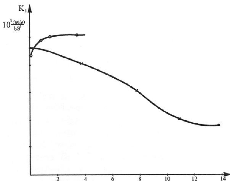
ნახ.1. Fe-X (X=Ni, Ti) შენადნობებში K_1 კონსტანტას დამოკიდებულება X-ის პროცენტულ შემცველობაზე
