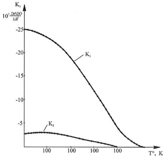
ნახ. 3. K_1 K_2 კონსტანტების ტემპერატურული დამოკიდებულება Y_3Fe_5O_{12} -ზე ლიტერატურა:
