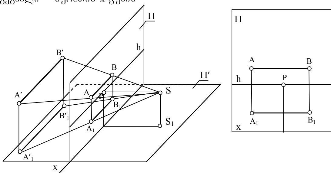
ნახ. 59 სურათის ფუძის პარალელური წრფის პერსპექტივა
