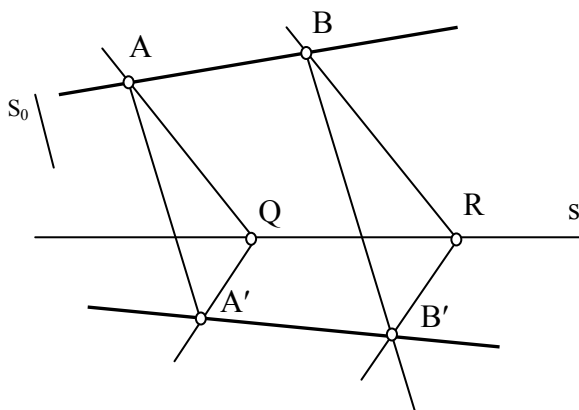
ნახ. 30 პერსპექტიულ-აფინური შესაბამისობა
