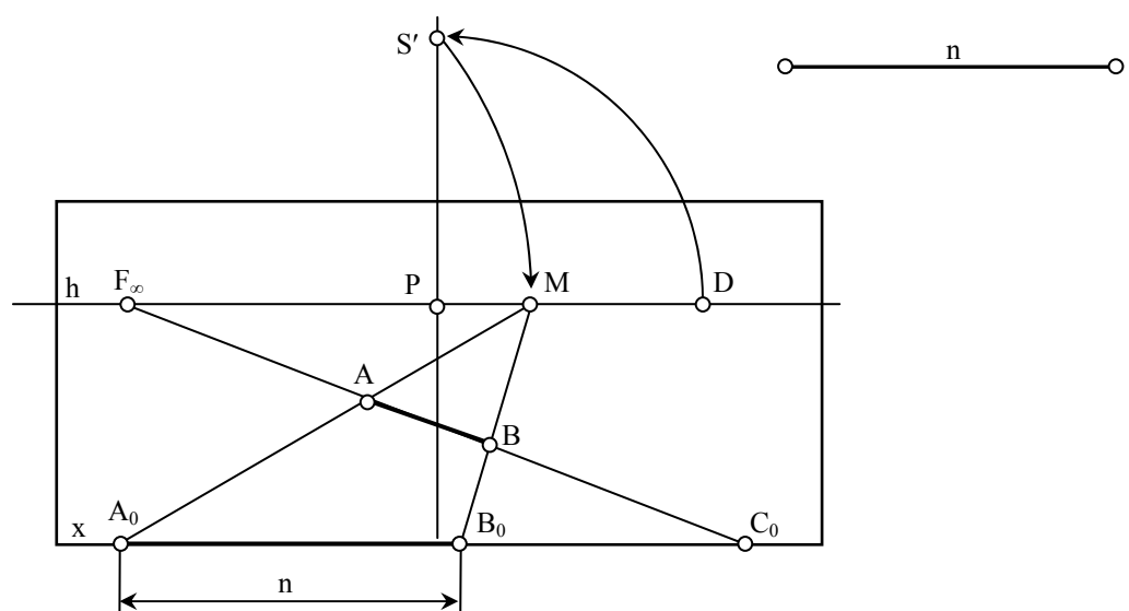
2) სურათზე მოცემულ წრეზე წინასწარ განსაზღვრული სივრცის მონაკვეთის აგება.
