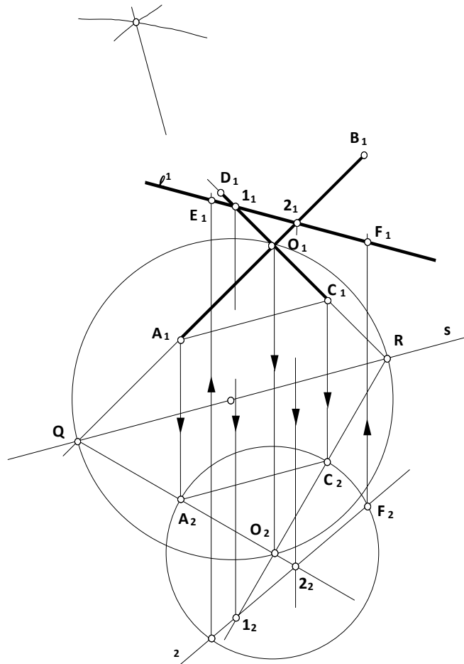
ნახ. 103 აფინურად შესაბამისი კვლების მთავარი მიმართულებები
