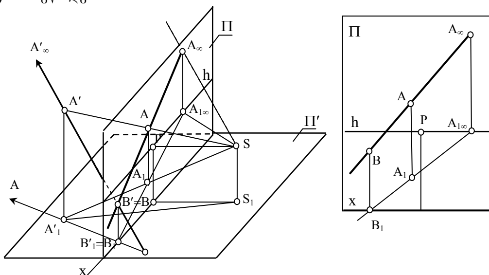
ნახ. 52 წრფის პერსპექტივა
