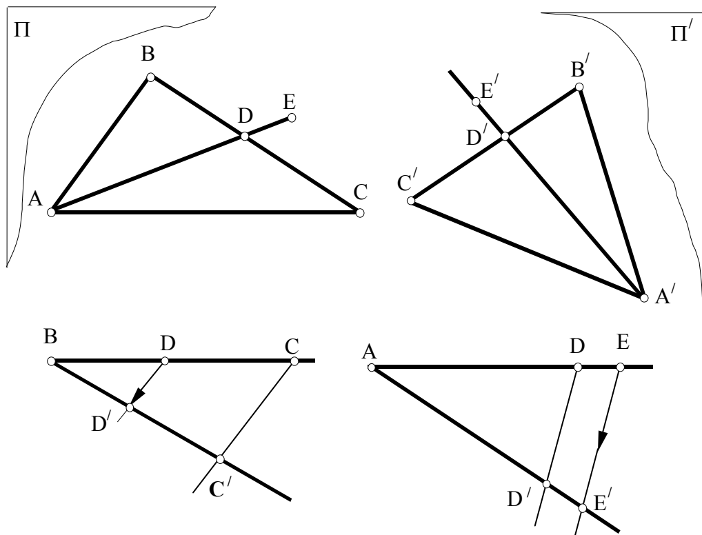
ნახ. 34 აფინური შესაბამისობა
