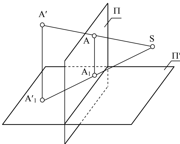
ნახ. 50 პერსპექტივის აპარატი
