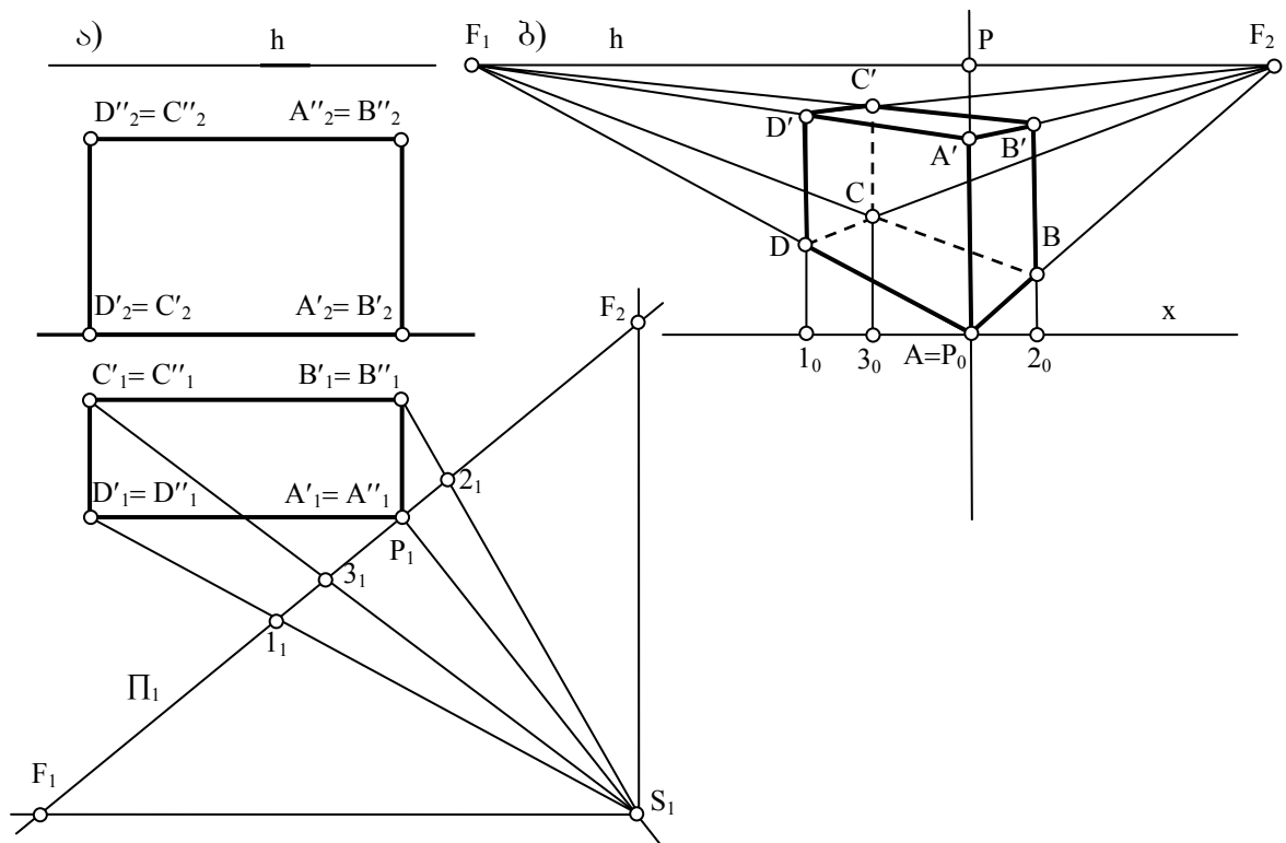
ნახ. 70 არქიტექტორების მეთოდი
