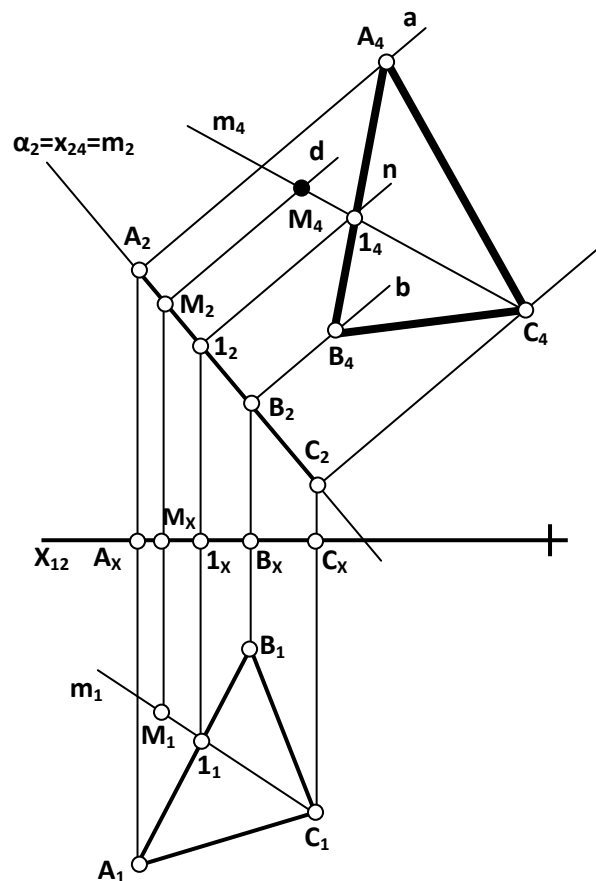
თუ მოცემულია M_1 წერტილი, რომელიც A_1B_1C_1 ბრტყელი ველის კუთვნილია, ცალსახად შეგვიძლია განვსაზღვროთ A_4B_4C_4 ბრტყელი ველის კუთვნილი და M_1 -ის შესაბამისი M_4 წერტილი. ჩვენ შემთხვევაში
