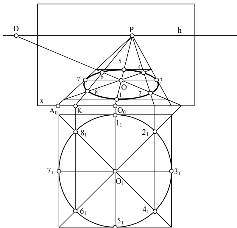
ნახ. 64 შემოსახული კვადრატის მეთოდი
