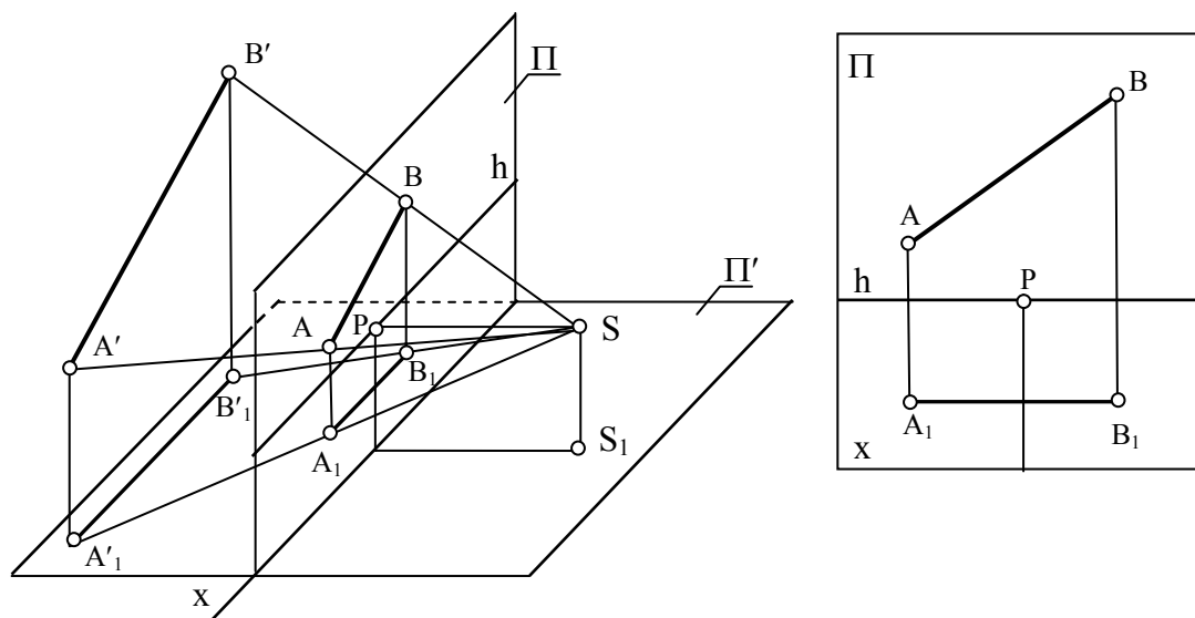
ნახ. 58 სასურათე სიბრტყის პარალელური წრფის პერსპექტივა
