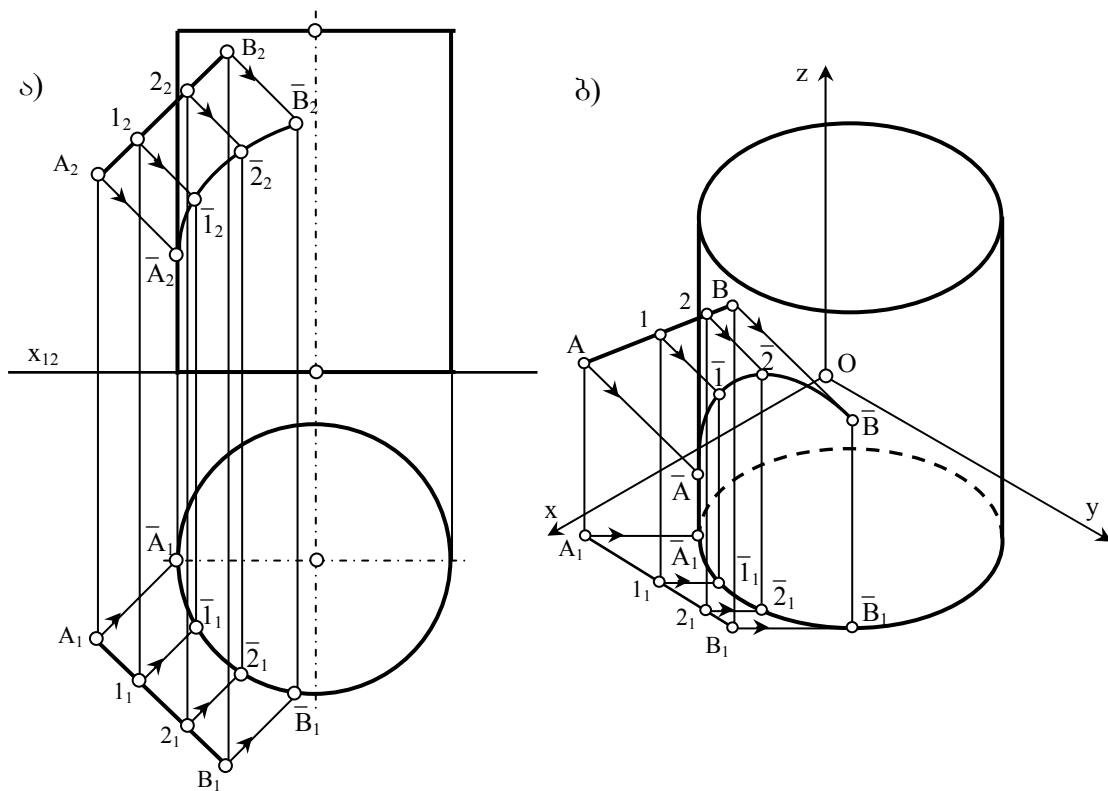
ნახ. 87 წრფის ჩრდილი მრუდ ზედაპირზე
