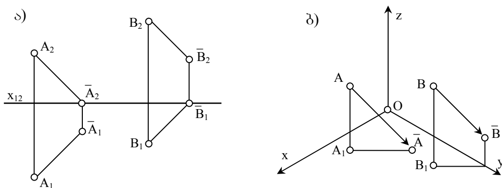
ნახ. 78 წერტილის ჩრდილი
