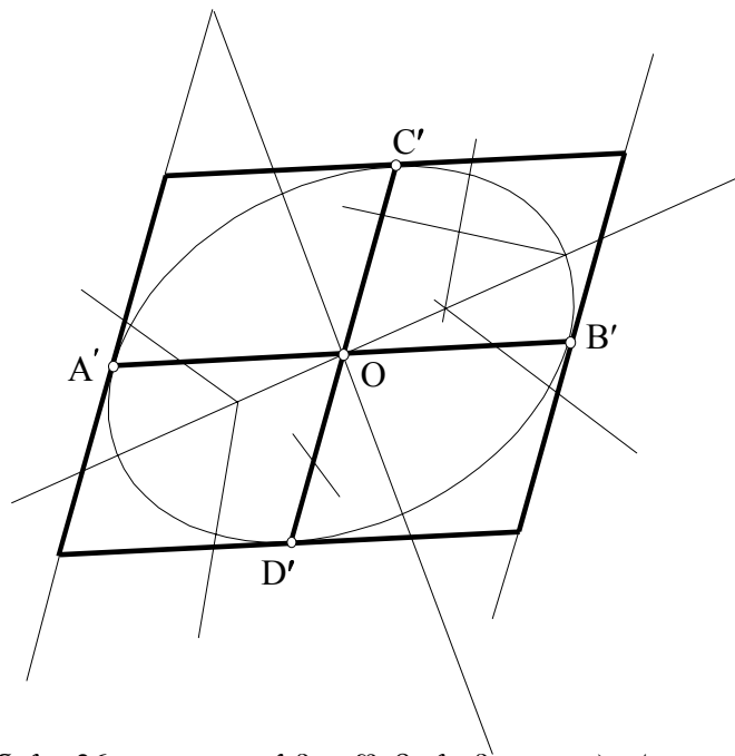
ნახ. 36 ელიფსზე შემოხაზული პარაბელოგრამი
