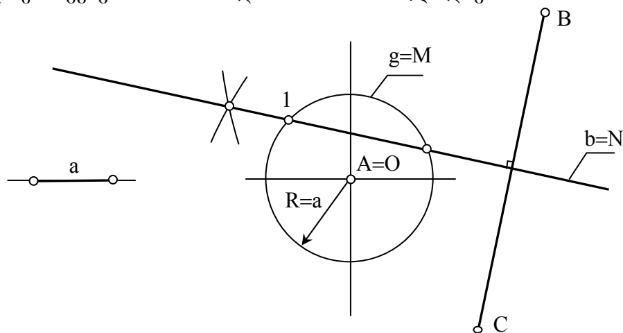
ნახ. 9 A წერტილიდან a მანძილით, ხოლო B და C წერტილებიდან ტოლი მანძილებით დაშორებული წერტილის აგება.
