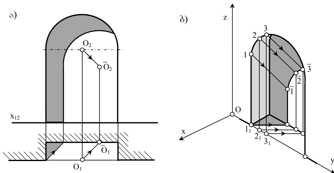
ნახ. 100 წრიულ ნიშაში დაცემული ჩრდილი
