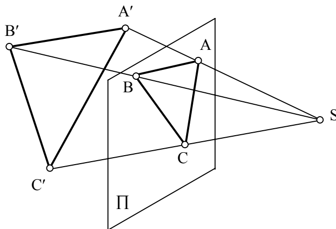
ნახ. 49 სამკუთხედის ცენტრალური გეგმილი
