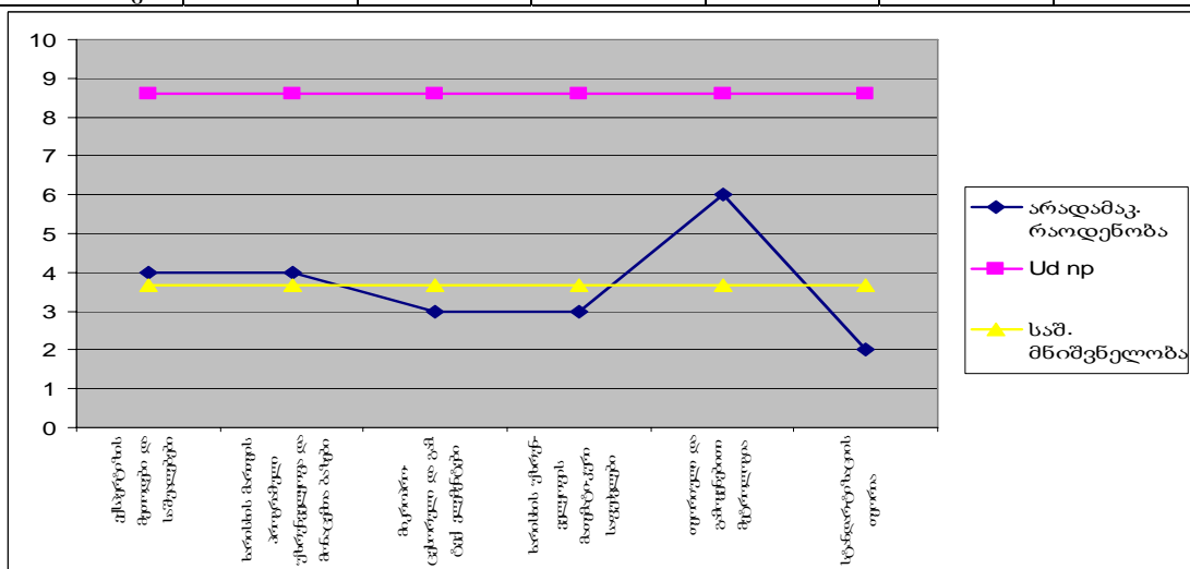
ნახ. 7. NP –საკონტროლო რუკა
