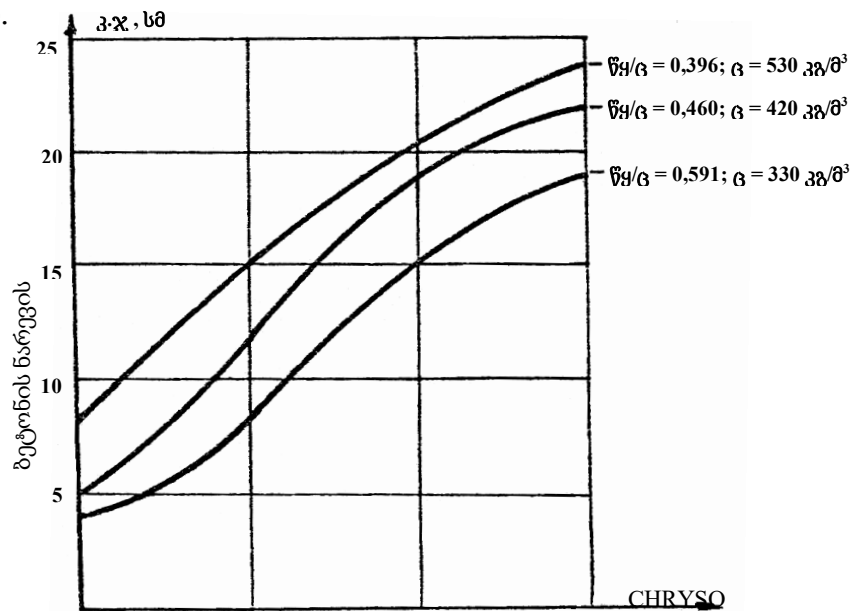
ნახ. 1. სუპერპლასტიფიკატორის ხარჯის დადგენა ბეტონის ნარევის დასახული ძვრადობის მისაღებად სხვადასხვა წ/ც-ისა და ცემენტის ხარჯისას
