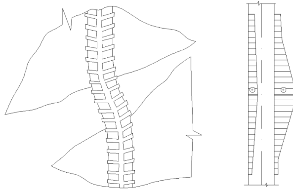
ნახ. 5 განივი არმატურის დეფორმირების საერთო სურათი და მისი განაწილება ღეროს სიგრძეზე.
