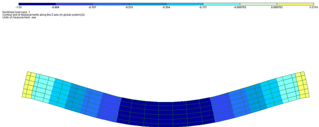
ნახ.12 რკინაბეტონის კოჭი (მმ)
