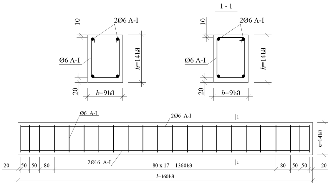
ნახ.7 რკინაბეტონის კოჭის განივი და გრძივი კვეთები
