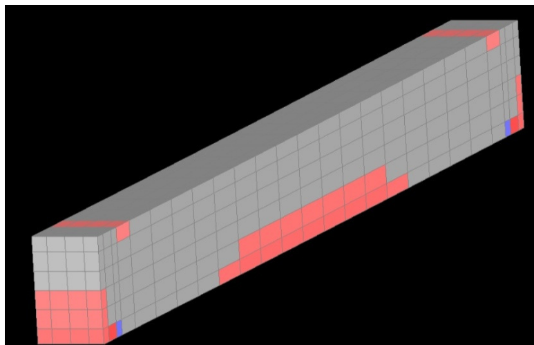
ნახ. 15. რკინაბეტონის კოჭის რღვევის სტადია
