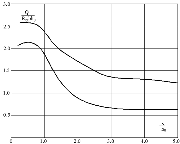
ნახ. 3 რკინაბეტონის ელემენტის ზიდვის უნარი ჭრის მაღის სხვადასხვა მნიშვნელობისათვის.
