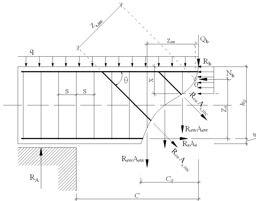
ნახ. 1 რკინაბეტონის კოჭში განივ ძალებზე განგარიშების საანგარიშო სქემა
