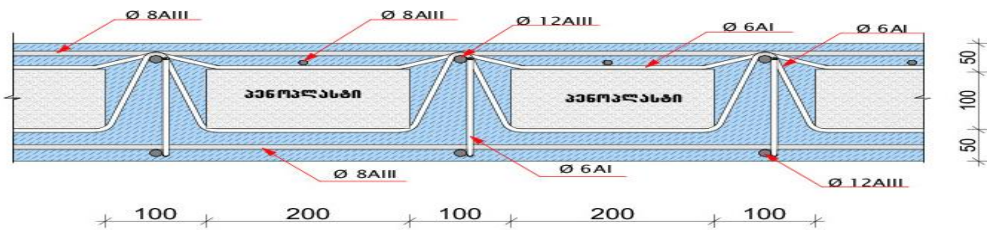
ნახაზი 6 არმატურის კარკასიანი თბოიზოლირებული გადახურვის ფილის განივი კვეთის სქემატური გამოსახულება.
