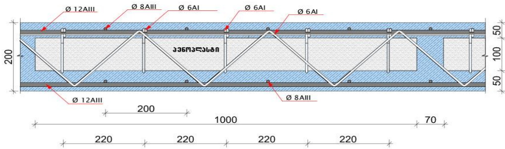
ნახაზი 5 არმატურის კარკასიანი თბოიზოლირებული გადახურვის ფილის გრძივი კვეთის სქემატური გამოსახულება
