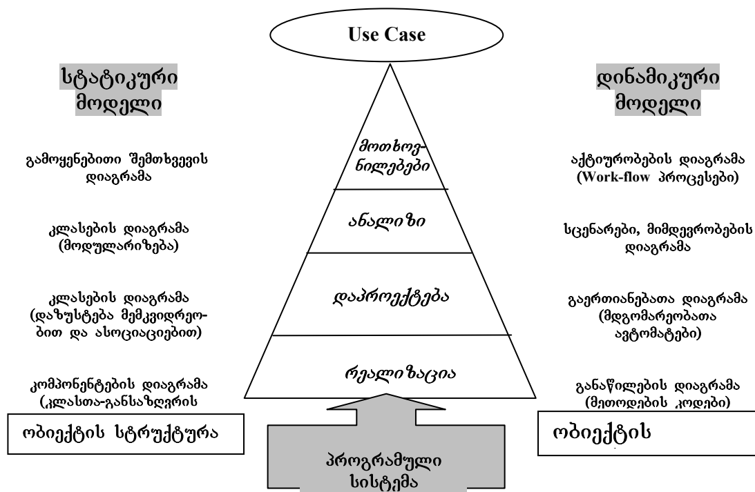
ნახ.2.3. სტატიკური და დინამიკური მოდელები
