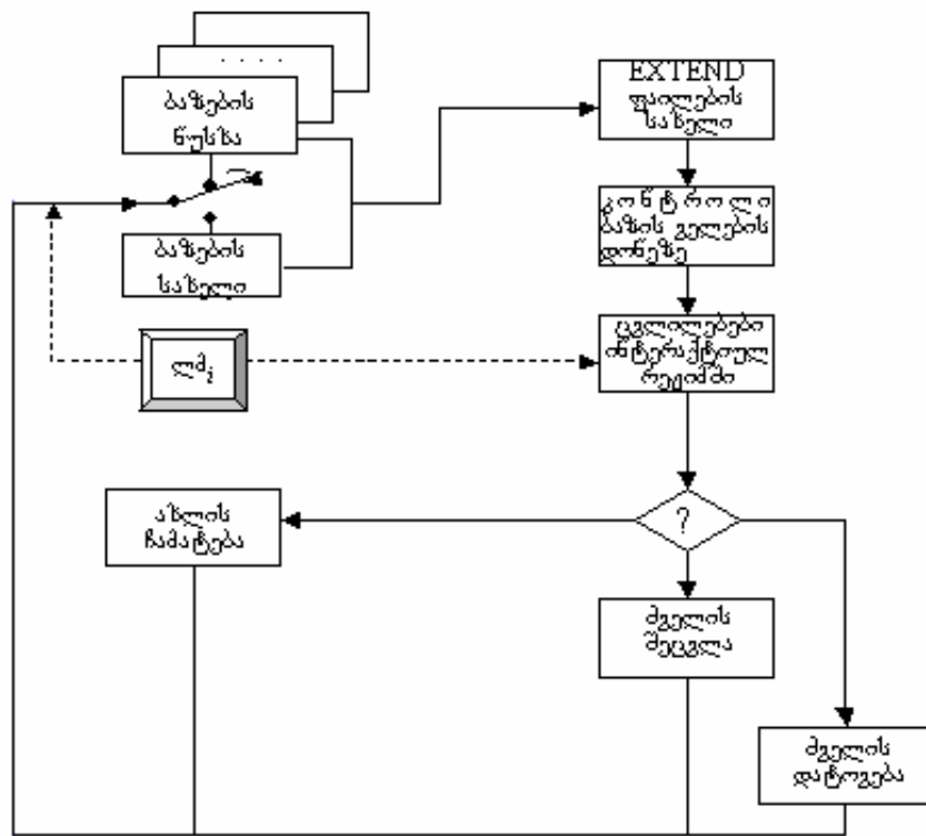
ნახ.3.7. მზის მთლიან მდგომარეობაში გადაყვანის ალგორითმი
