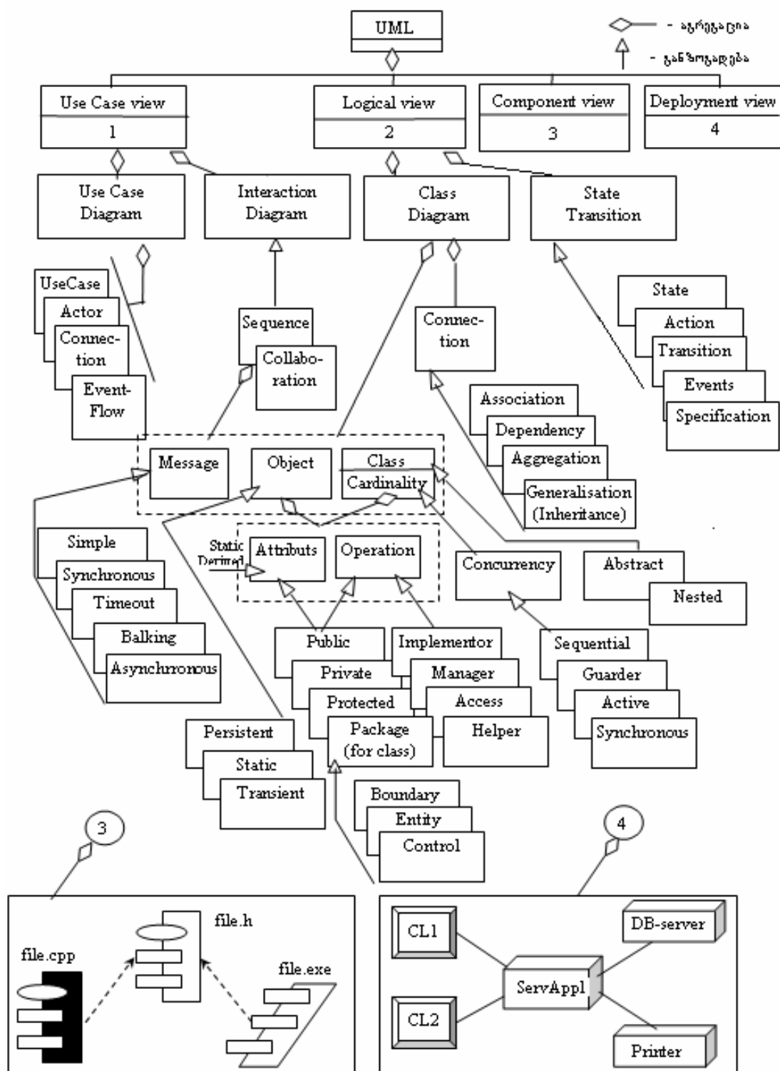
ნახ.2.4. UML სტრუქტურა Rational Rose მაგალითზე
