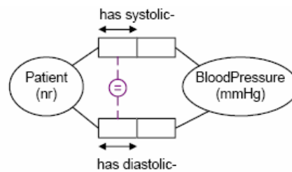
ნახ.2.21. ტოლობის შეზღუდვა
