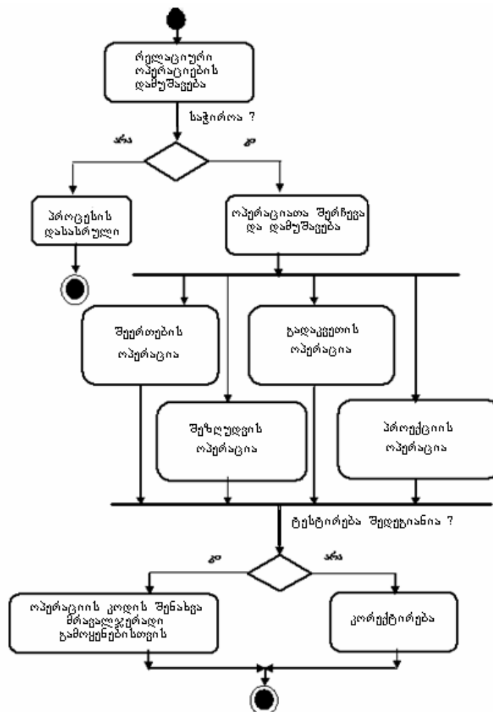
ნახ.2.10. მბ-ის რელაციური ოპერაციების დამუშავების პროცესის აქტიურობის დიაგრამა
