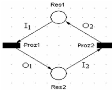
ნახ.2.15. ჩიხური სიტუაციის მაგალითი
