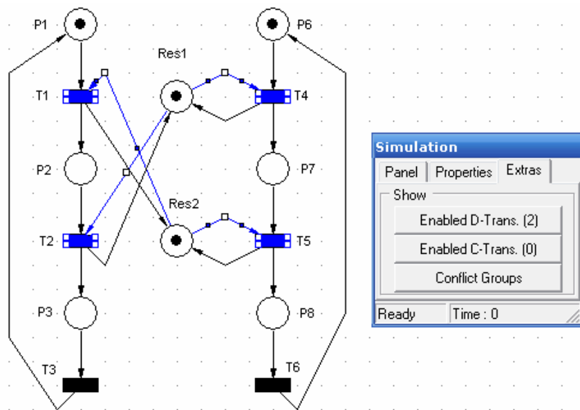
ნახ.2.17. კონფლიქტური ჯგუფის გადასასვლები
