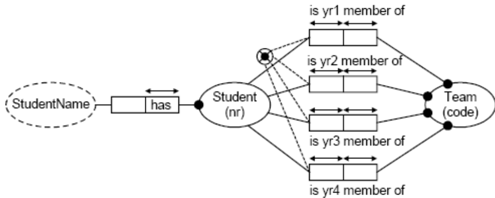
ნახ.2.28. იძულების დიზუნქციის შეზღუდვა (მაგ.3)
