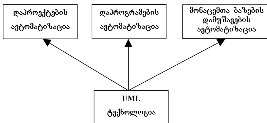
ნახ.2.1. UML ტექნოლოგიის კონცეფცია
