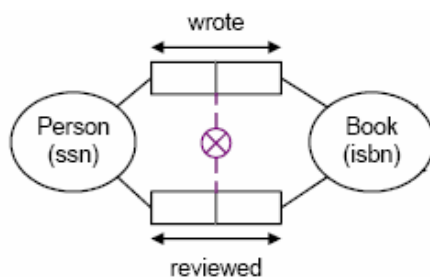
ნახ.2.22. წვილის გამორიცხვის შეზღუდვა (მაგ.1)
