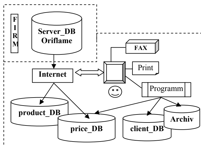
ნახ.3.3. შპსს-ს სტრუქტურა
