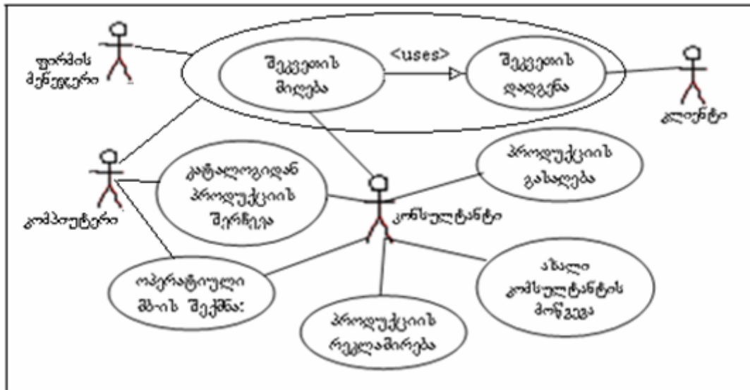
ნახ.3.1. UseCase დიაგრამის ფრაგმენტი
