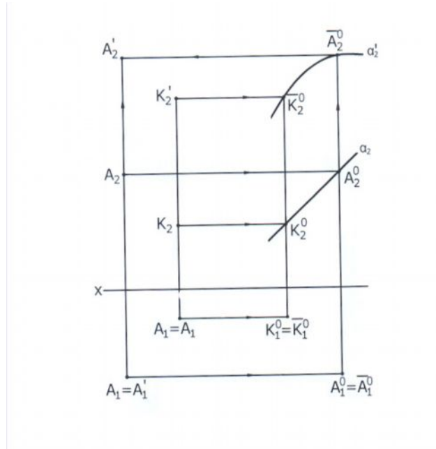
ნახ. 6. შესაბამისი წერტილის აგების გრაფიკული სქემა.
