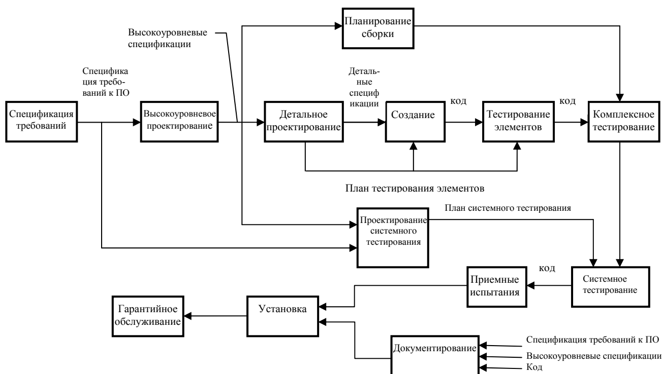
Рис. 3. Процесс разработки программного обеспечения.
