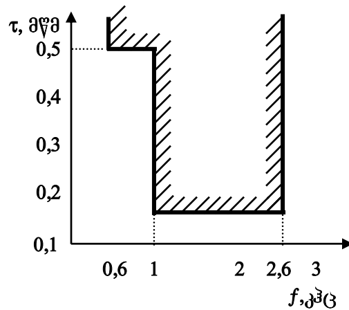
სურ. 2.8. ციფრული ტს-ს არხის ბჰდ-ს დასაშვები არათანაბრობის შაბლონი
