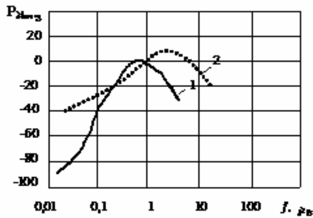
სურ. 114. პსოფომეტრული ფილტრის სიხშირული მახასიათებელი: 1 – სატელეფონო კავშირისათვის; 2 – ზუწყებლობისათვის
