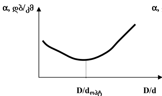
სურ. 3.3. კოაქსიალური კაბელის მიღევის კოეფიციენტის დამოკიდებულება გამტარების დიამეტრების ფარდობაზე
