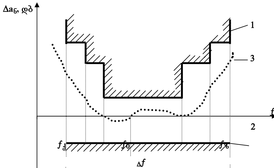
სურ. 2.2. ნარჩენი მიღევის ნომინალური მნიშვნელობიდან გადახრების შაბლონის სანიმუშო სახე: f_0 – სიხშირე, რომელზეც განისაზღვრება ნარჩენი მიღევის ნომინალური მნიშვნელობა; f_k, f_{kx} – ეფექტურად გადაცემული სიხშირეთა ზოლის ქვედა და ზედა საზღვრები; 1, 2 – ნარჩენი მიღევის დასაშვები გადახრების საზღვრები; 3 – ნარჩენი მიღევის გაზომილი სიხშირული მახასიათებლის სახე
