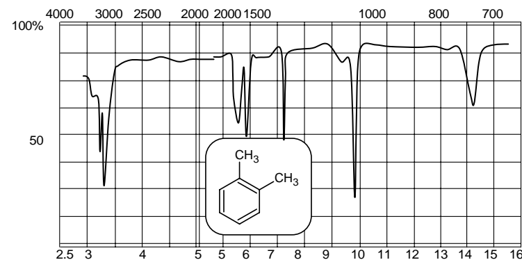
ნახ. 11. არომატული ნაერთების იწ სპექტრები: ბენზოლი, 1,2-დიმეთილბენზოლი
