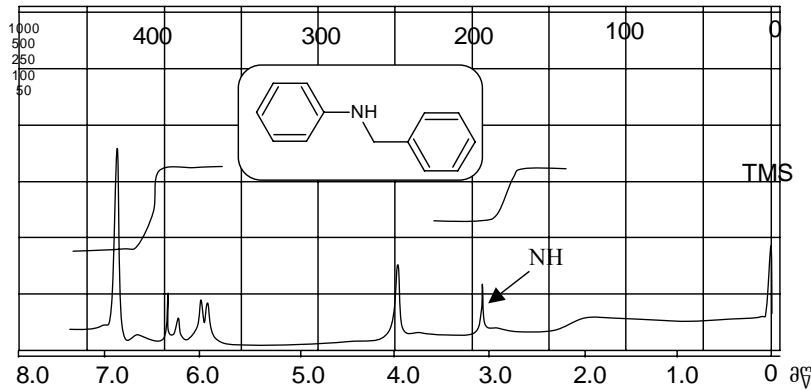
ნახ. 47. ფენილეთანამინის H 1 -ბმრ სპექტრი
