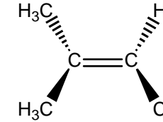
2-მეთილ-1-ქლორპროპენი
