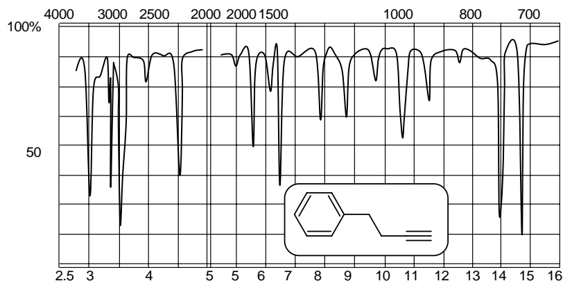
ნახ. 9. 5-ფენილ-1-ჰენტინის იწ სპექტრი
