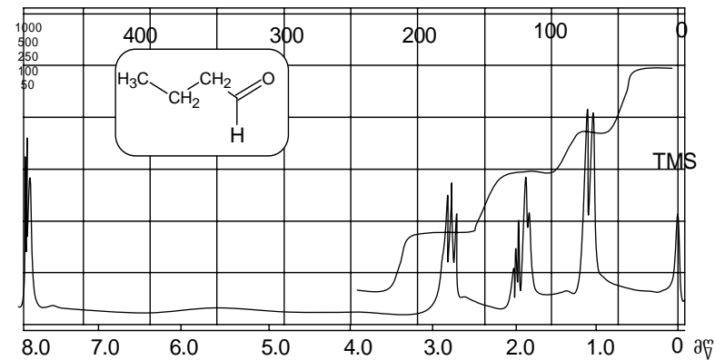
ნახ. 41. ბუტანალის H^1 -ბმრ სპექტრი
