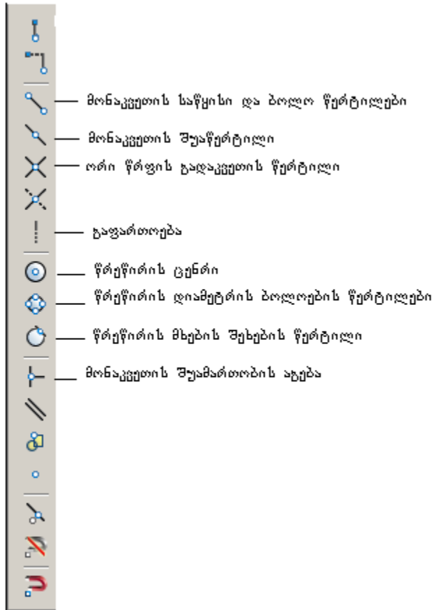
ნახ. 4. 11.Object Snap -ის ღილაკები.
