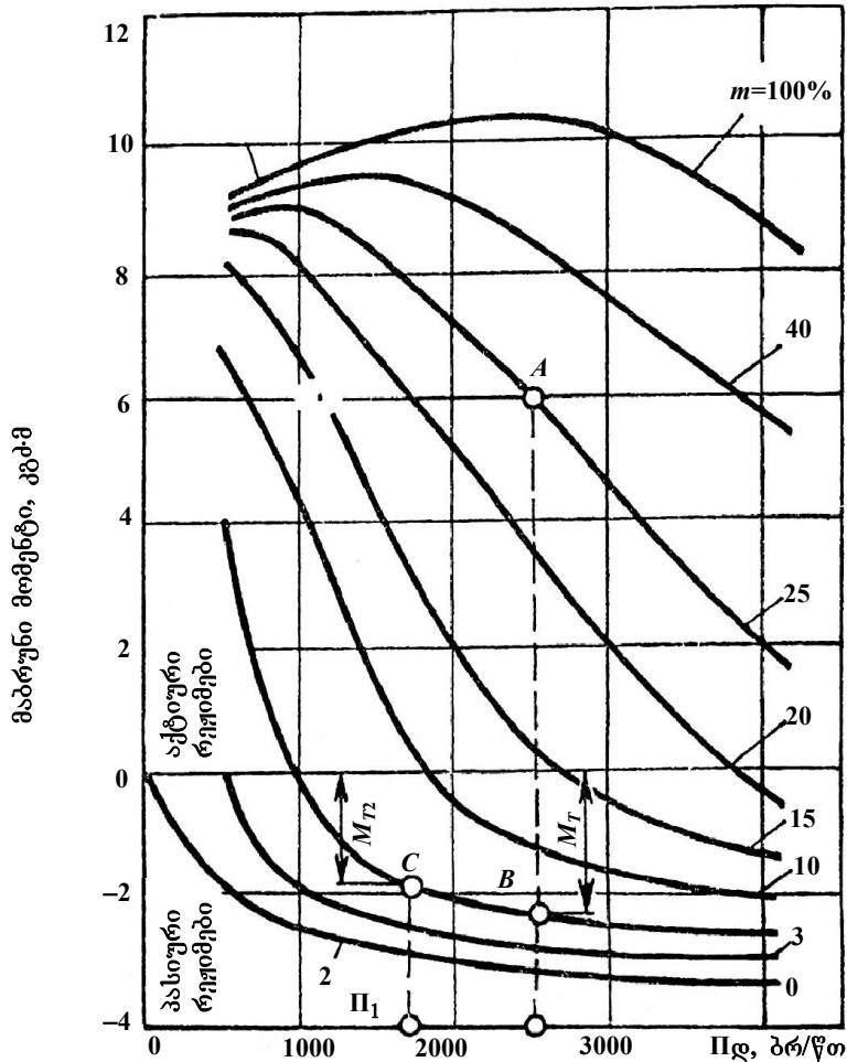
ნახ. 3.12. ავტომობილის ძრავის სიჩქარული და სამუხრუჭო მახასიათებლები
