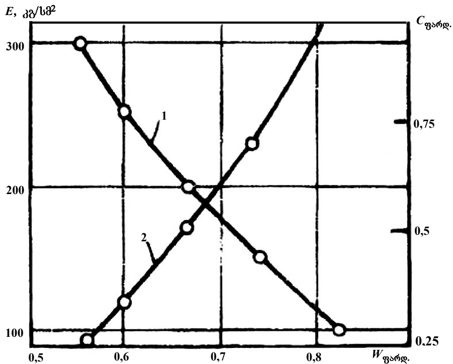
ნახ. 7.3. საგზაო სამოსის საფუძველი გრუნტის ტენიანობის გავლენა მის დეფორმაციის მოდულზე და საგზაო სამოსის ფარდობითი ღირებულება.
