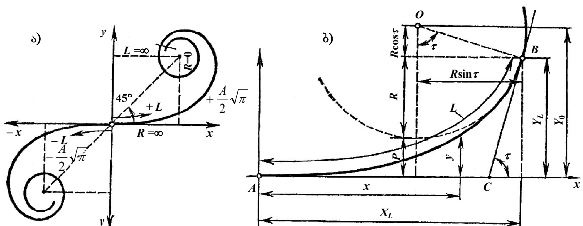
ნახ. 4.10. კლოტიდური გადასასვლელი მრუდი ა - კლოტიდა; ბ - სწორი და წრიული მრუდის შეერთება კლოტიდით.
