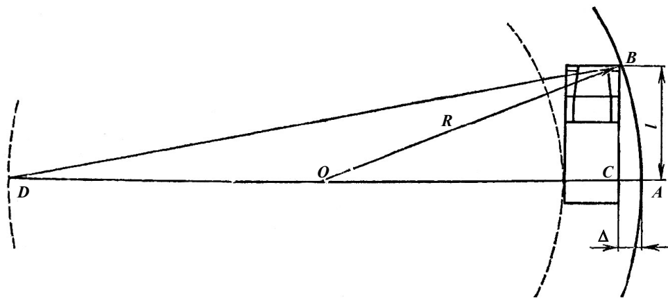
ნახ. 4.12. მრუდზე სავალი ნაწილის სიგანის საანგარიშო სქემა.
