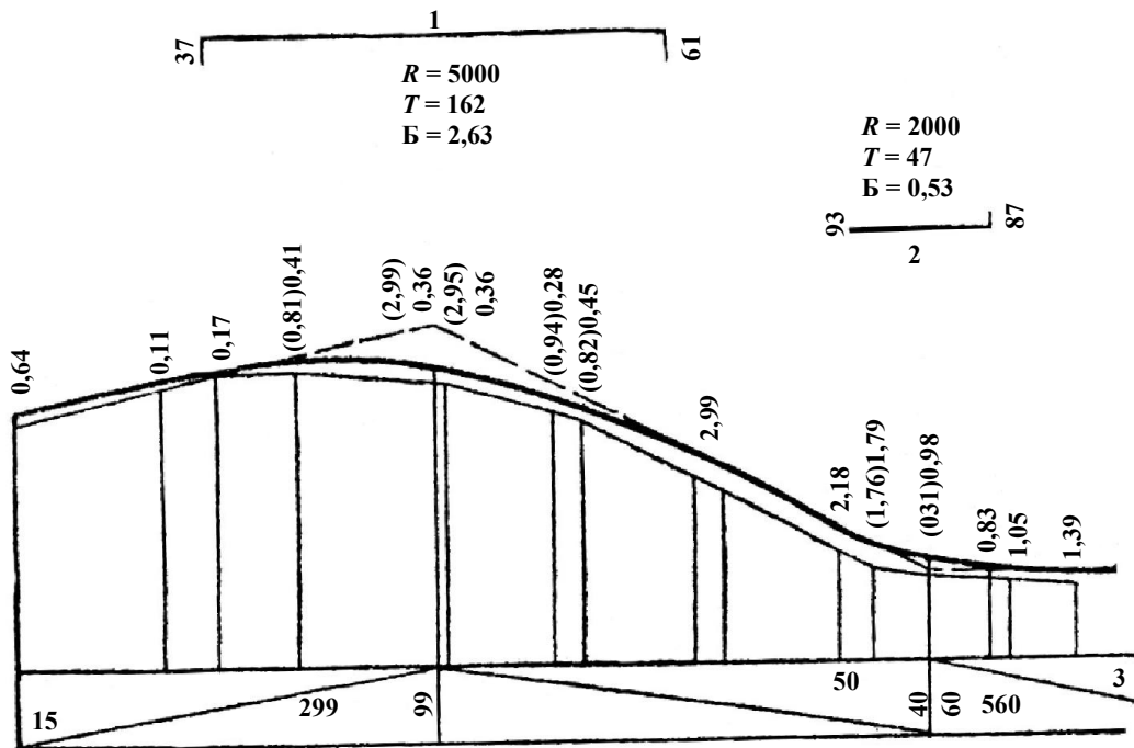
ნახ. 2.6. ვერტიკალური მრუდები: 1 - ამოზნექილი; 2 - ჩაზნექილი
