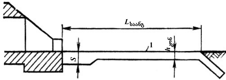
ნახ. 9.14. ნაგებობის იქით გამაგრების გრძივი ჭრილი.
