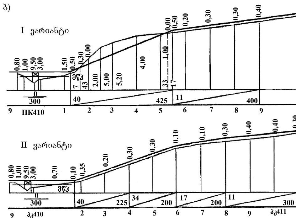
ნახ. 10.6. ფერდობზე ტრასის განლაგების ვარიანტები: ა - გეგმა; ბ - გრძივი პროფილი.
