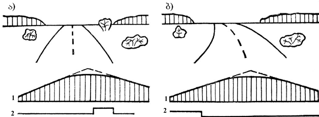
ნახ. 12.11. მძლოლის მხედველობითი ორიენტირების გაუმჯობესება: ა - გზის ხიდი მხედველობითი სიძლიერის პრინციპის დარღვევით; ბ - გზის ხედის გაუმჯობესება ჰორიზონტალური მრუდის სიგრძის გაზრდით; 1 - გრძივი პროფილი; 2 - გეგმა.
