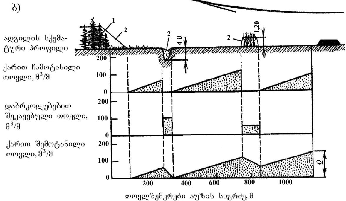
ნახ. 10.4. სქემა გზაზე შემოსული თოვლის რაოდენობის განსაზღვრისათვის: ა – თოვლის დამგროვებელი აუზის გეგმა; ბ – სქემა ჩამოტანილი და შეკავებული თოვლის განსაზღვრისათვის; 1 – ტყის პირი; 2 – აეროდინამიკური ჩრდილის საზღვრები.
