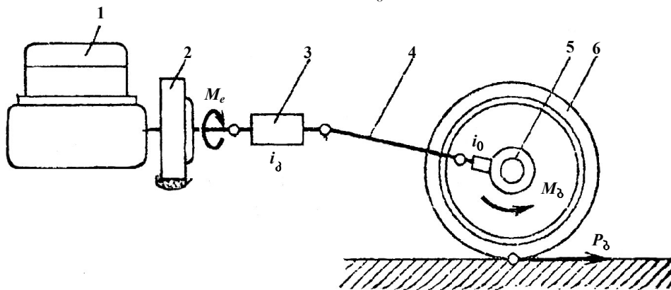
ნახ. 3.4. ძრავის მაბრუნე მომენტის გადაცემის სქემა ავტომობილის თვლებზე: 1 – ძრავი; 2 – გადაბმის ქურო; 3 – სიჩქარის კოლოფი; 4 – კარდანის დერძი; 5 – მთავარი გადაცემა; 6 – საბურავი.
