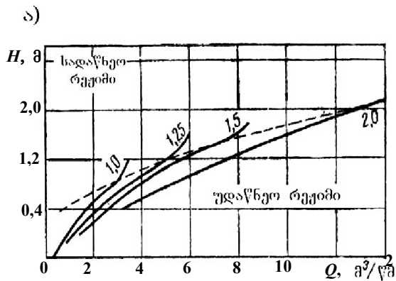
ნახ. 9.6. ტიპური უნიფიცირებული მილების გამტარუნარიანობის გრაფიკები: ა – მრგვალი მილებისათვის; ბ – სწორკუთხა მილებისათვის, ციფრები მრუდებზე - მილის ხერცები, მ
