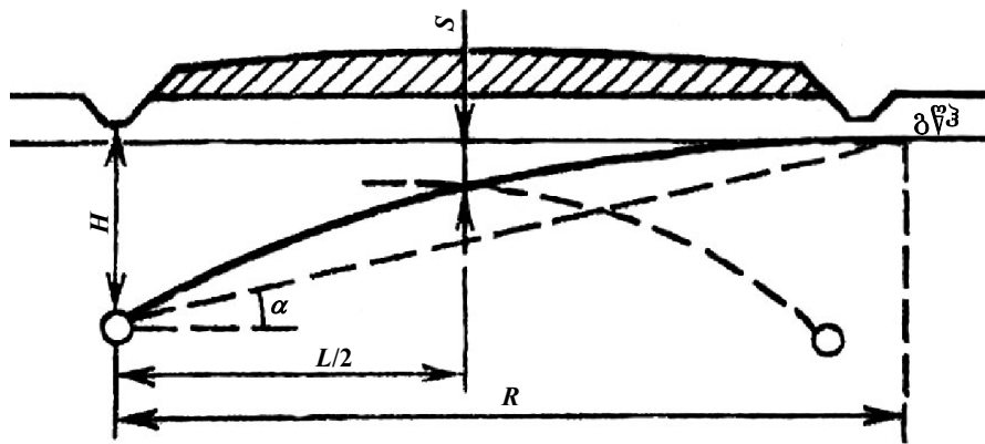
ნახ. 8.13. კოეფიციენტის ქვედა დრენაჟის საანგარიშო სქემა.
