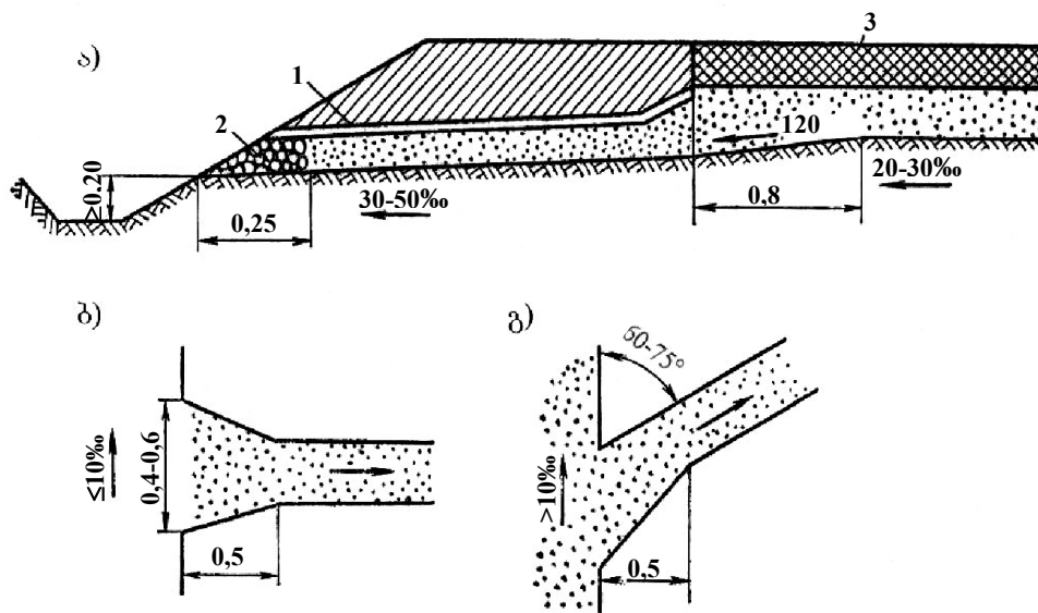
ნახ. 8.9. სადრენაჟო დაბრუნი:
