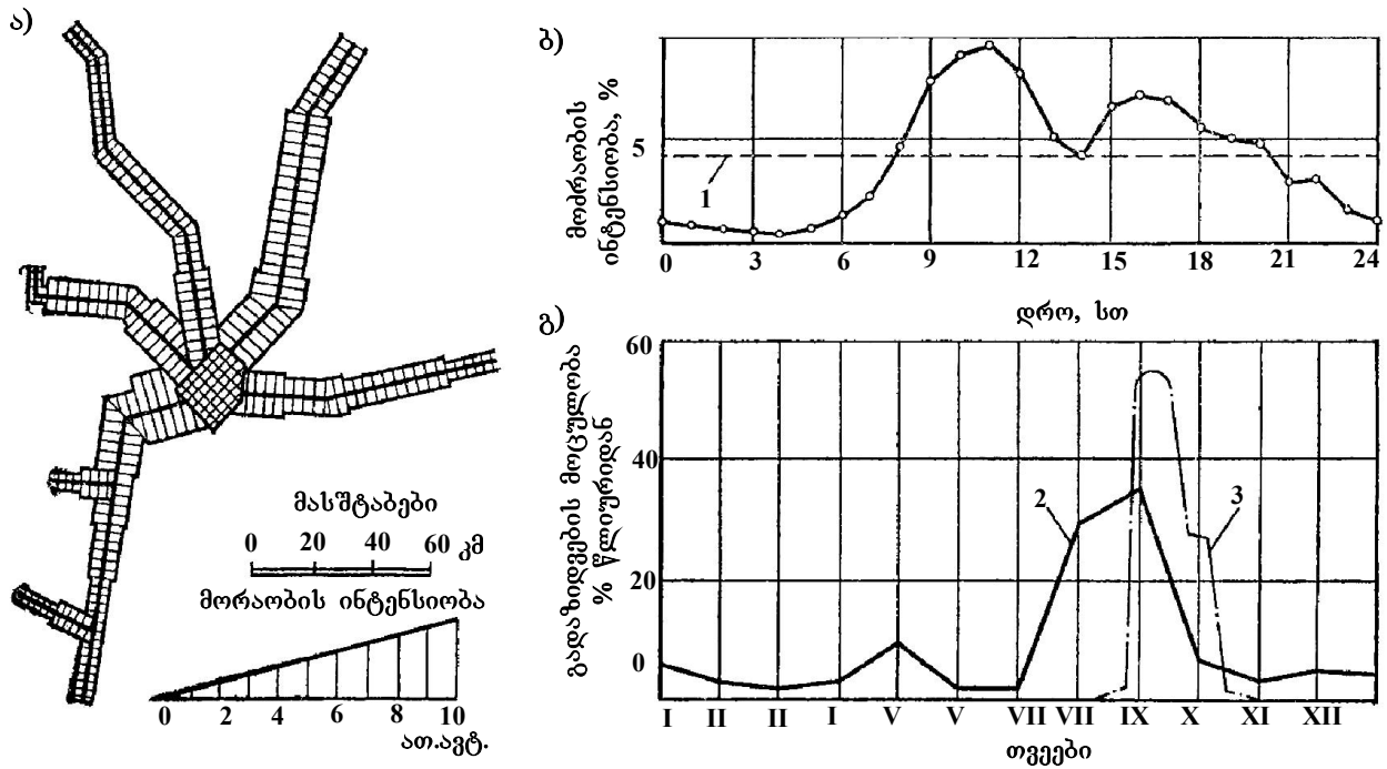
ნახ. 12. მოძრაობის ინტენსიობის ცვლილება მისასვლელი გზის სხვადასხვა უბანზე ა), დღელამის განმავლობაში ბ) თვეების მიხედვით გ)
