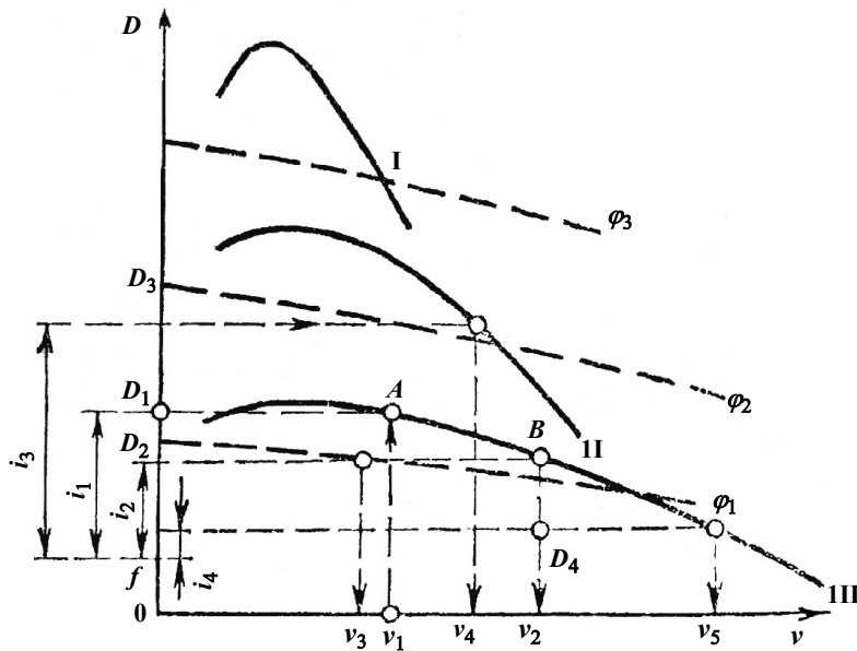
ნახ. 3.9. დინამიურ მახასიათებელთა გრაფიკი წვევის ანგარიშებისათვის
