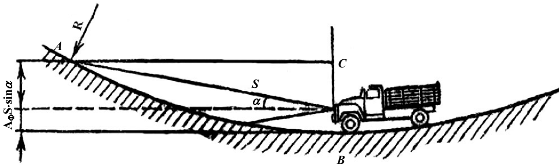
ნახ. 5.4. მხედველობა ჩაზნექილ მრუდზე ავტომობილის ფარების განათებისას
