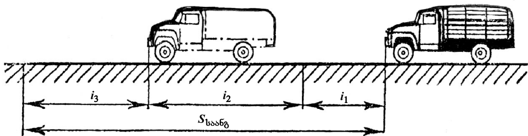
ნახ. 3.11. სამუხრუჭო მანძილის საანგარიშო სქემა S – საანგარიშო სამუხრუჭო მანძილი; l_1 – რეაქციის პერიოდში გავლილი მანძილი; l_2 – სამუხრუჭო მანძილი; l_3 – უსაფრთხოების მანძილი
