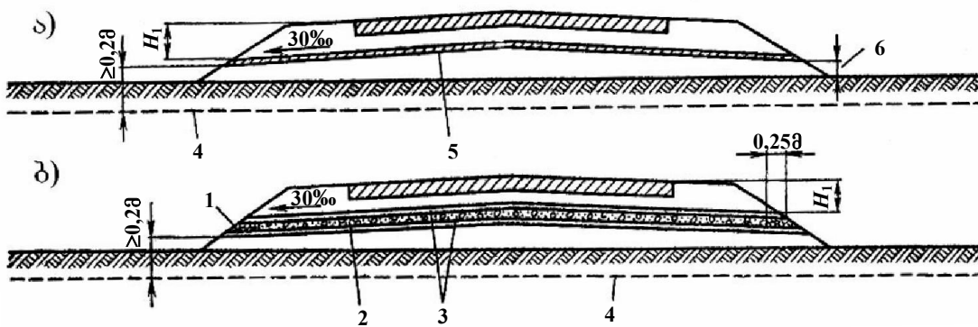
ნახ. 7.5. მიწის ვაკისის ფენები:
