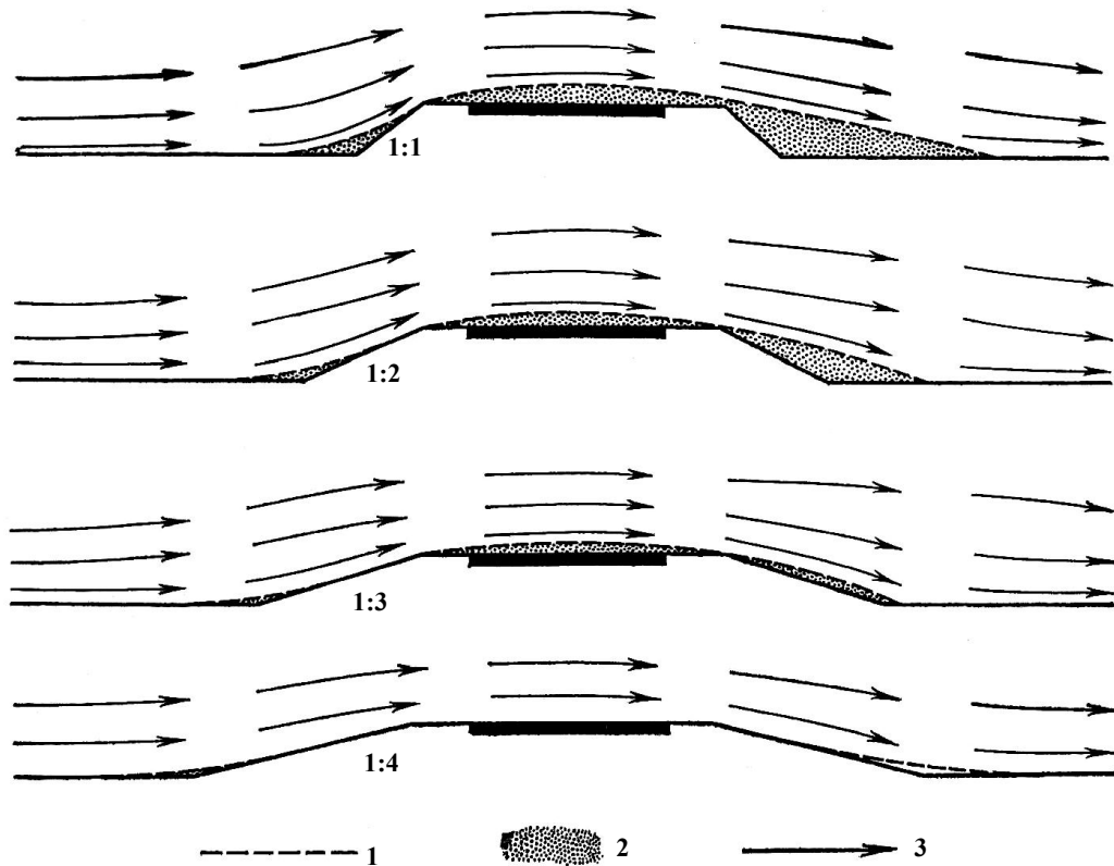
ნახ. 2.11. ყრილის ფერდობების დახრილობის გავლენა მიწის ვაკისის ქარბუქისაგან დაცვაზე:
