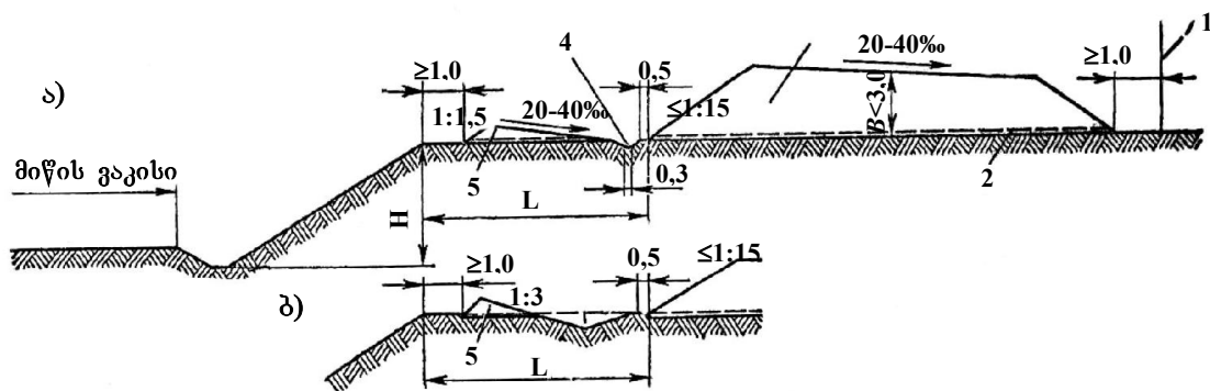
ნახ. 2.14. კავალიერების განლაგების სქემა:
