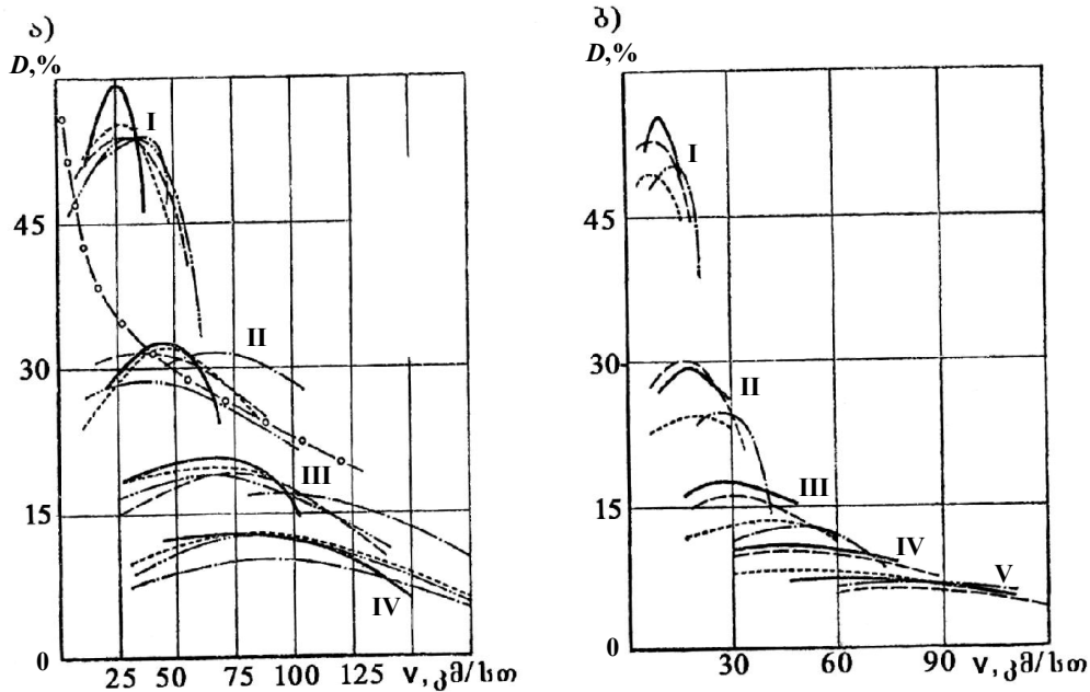
ნახ. 3.6. სხვადასხვა მარკის ავტომობილთა დინამიური მახასიათებლები. ა - მსუბუქი ავტომობილები; ბ - სატვირთო ავტომობილები.
