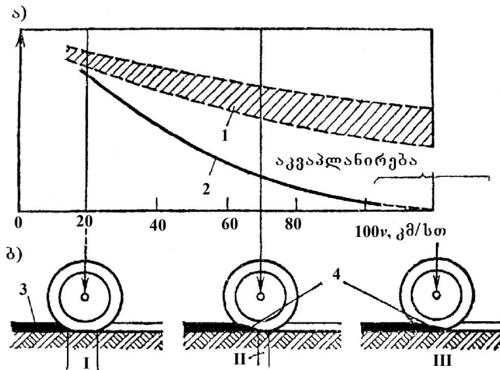
ა - შეჭიდულობის კოეფიციენტის ცვლილება სიჩქარისაგან გზის სველ ზედაპირზე; ბ - საბურავის კონტაქტის ზონის შემცირება გზის სველ ზედაპირთან სიჩქარის გაზრდის შედეგად; 1 - საბურავები ახალი პროტექტორით; 2 - გაცვეთილი საბურავები; 3 - წყლის აფსკი > 1 მმ; 4 - საბურავის ქვეშ წარმოქმნილი წყლის სოლი: I - ბორბლისა და ფენილის კონტაქტის მთლიანი ზონა; II - შემცირებული ზონა; III - კონტაქტი აღარაა.
