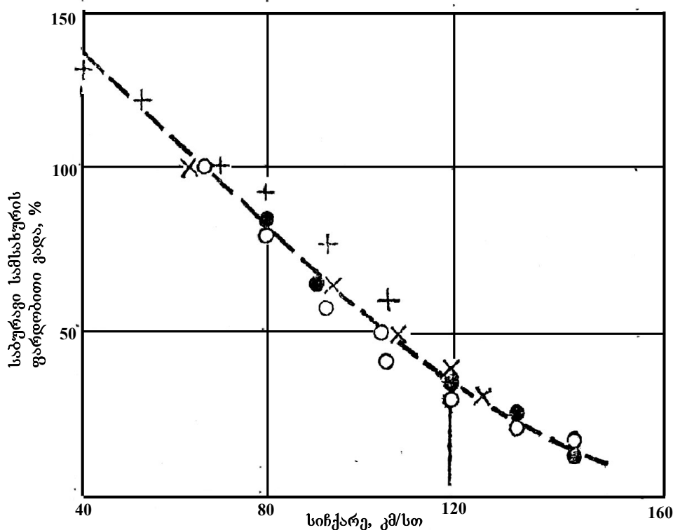
ნახ. 3.16. საბურავების ცვეთის დამოკიდებულება მოძრაობის სიჩქარისაგან (სხვადასხვა ავტორთა ექსპერიმენტული მონაცემები)
