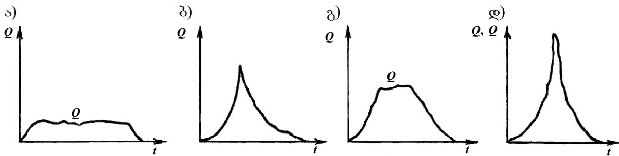
ნახ. 8.3. წყლის მოდინების გრაფიკები დროში:
