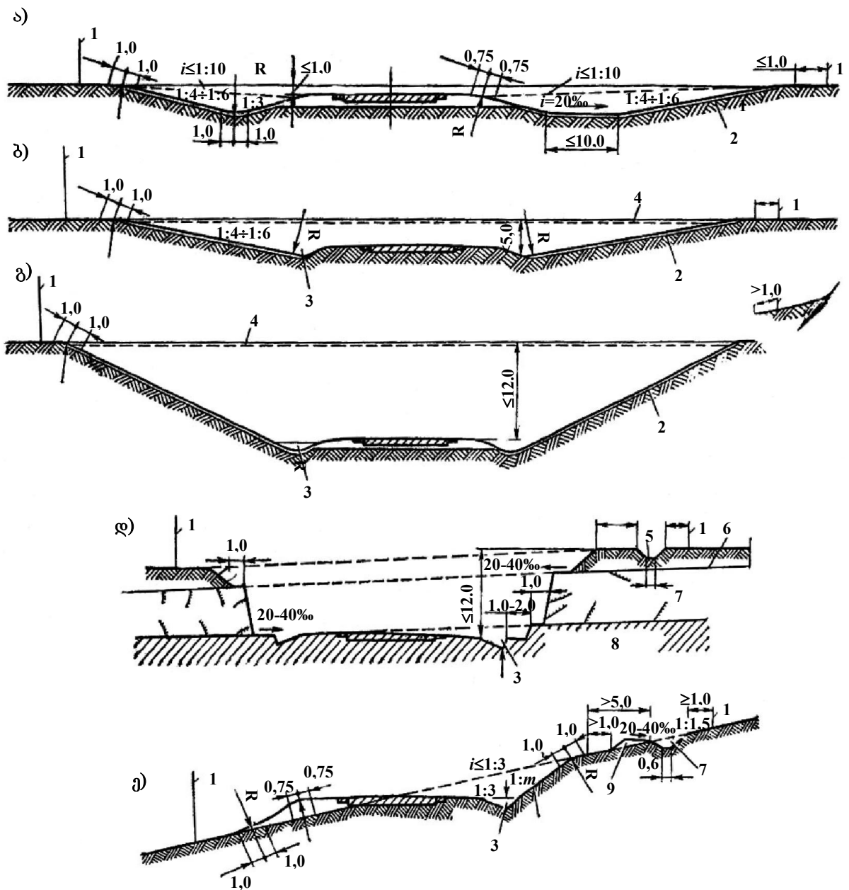
ნახ. 2.13. მიწის ვაკისის განივი პროფილები ჭრილებში:
