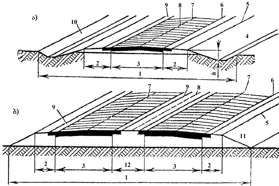
ნახ. 2.10. გზის განივი პროფილის ელემენტები:
