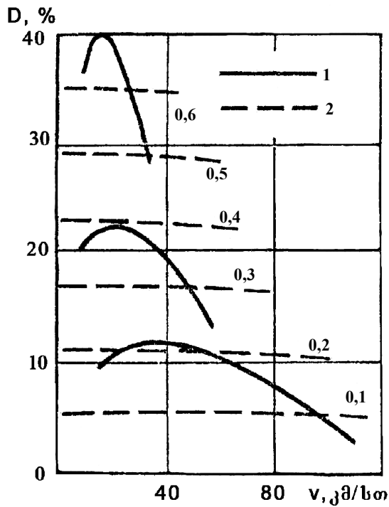
ნახ. 3.8. ავტომობილის დინამიური მასხასიათებელი შეზღუდვა შეჭიდულობით: 1 – წვევის ძალა; 2 – მისი შეზღუდვა შეჭიდულობით. ციფრები პუნქტირით დახაზულ მრუდებზე გვიჩვენებენ შეჭიდულობის კოეფიციენტის სიდიდეს.
