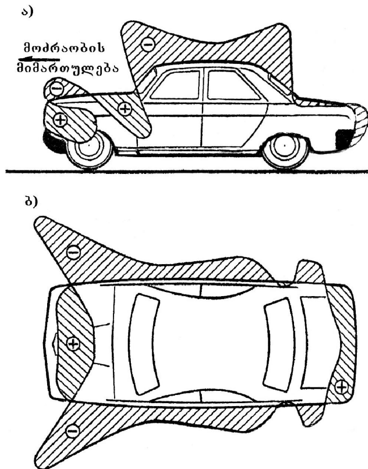
ნახ. 3.2. ჰაერის დაწნევის განაწილება მოძრავ ავტომობილზე: ა – დაწნევის ეპიურა სიმეტრიის ღერძის გასწვრივ ვერტიკალურ სიბრტყეში; ბ – დაწნევის ეპიურა ბუფერის დონის ჰორიზონტალურ სიბრტყეში.
