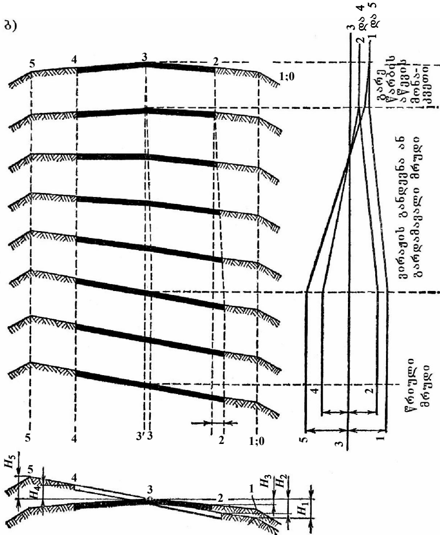
ნახ. 4.14. ორმხრივად დახრილი სავალი ნაწილიდან ცალმხრივ დახრაზე გადასვლის საშუალებები ა – განივი პროფილის აწევა გზის ღერძის ზემოთ; ბ – განივი პროფილის ბრუნება გზის ღერძის გარშემო; 1-5 განივი პროფილის მახასიათებელი წერტილები
