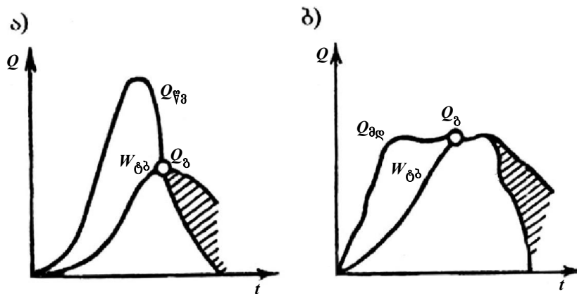
ნახ. 9.7. წყლის მიდინების ჰიდროგრაფის გარდაქმნა ნაგებობასთან. გადასაგდები ხარჯების ჰიდროგრაფად. ა – ნიაღვრის ჩამონადენი; ბ – მდნარი წყლების ჩამონადენი.
