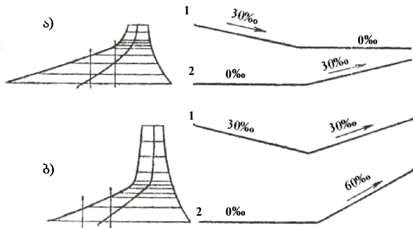
ნახ. 12.8. გრძივი პროფილის დამახინჯება პერსპექტივაში. ა – დახრილი მონაკვეთის შემდეგ კორიზონტალური აღიქმება, როგორც ადმართი; ბ – დახრილი მონაკვეთის შემდეგ მცირე ადმართი აღიქმება ციცაბო ადმართად.
