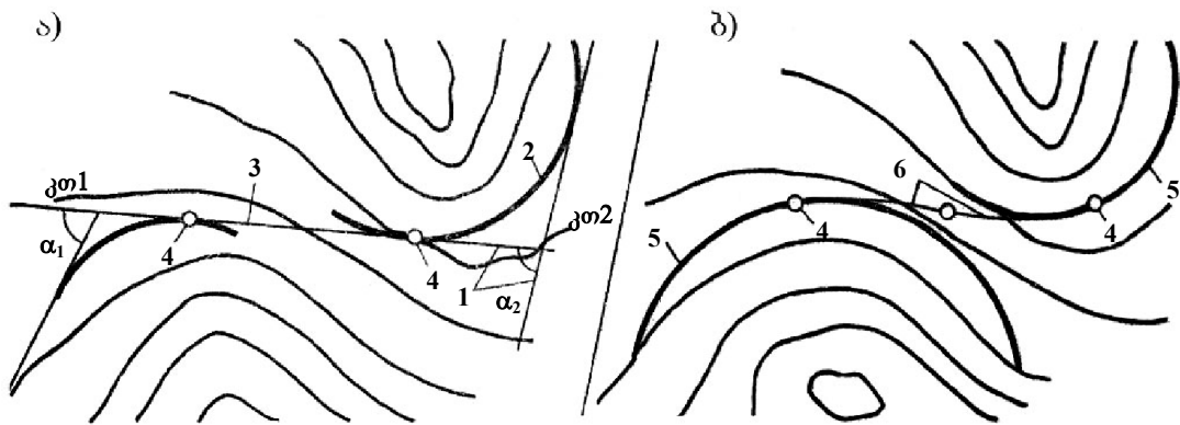
ნახ. 12.13. საავტომობილო გზების ტრასირების პრინციპების სხვაობა:
