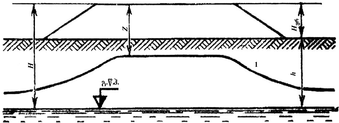
ნახ. 7.4. მიწის ვაკისის წარბას აწევის სქემა დატენიანების წყაროებიდან 1 – ზამთარში გაყინვის სიღრმე
