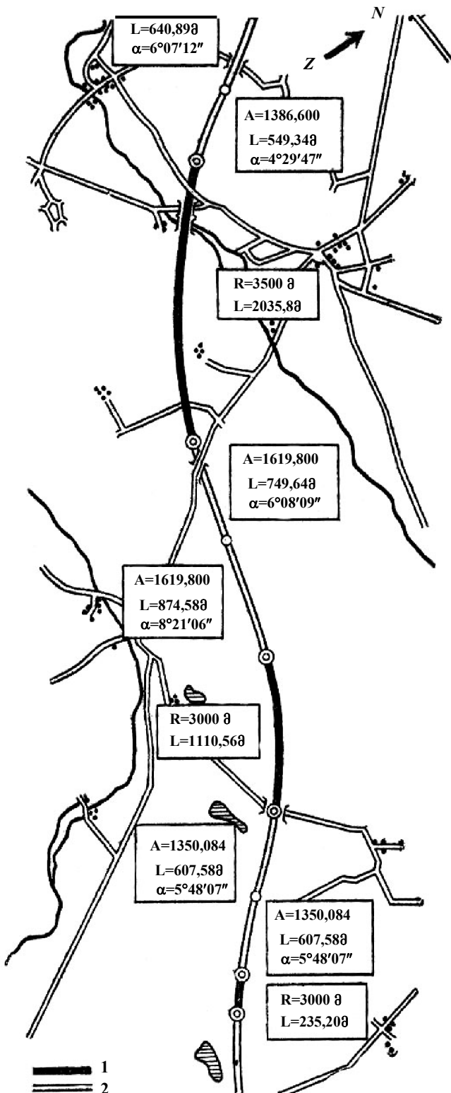
ნახ. 12.12. კლოტოიდებით ტრასირებული გზა:
