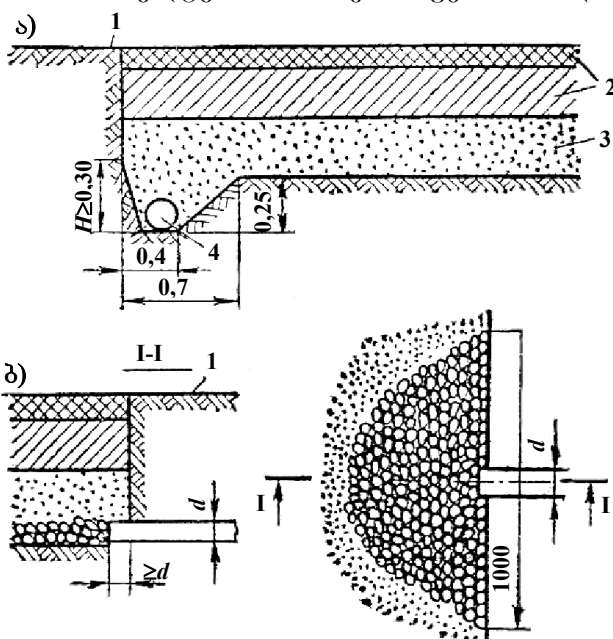
ნახ. 8.10. ქვიშის საფუძველის დასაშრობი სადრენაჟო მილები:
