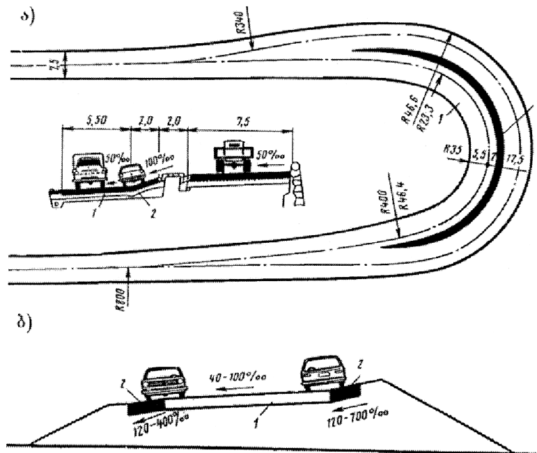
ნახ. 4.17. მოძრაობის პირობების გაუმჯობესება მკვეთრ მოსახვევებში საფეხურიანი ვირაუის მოწყობით:
