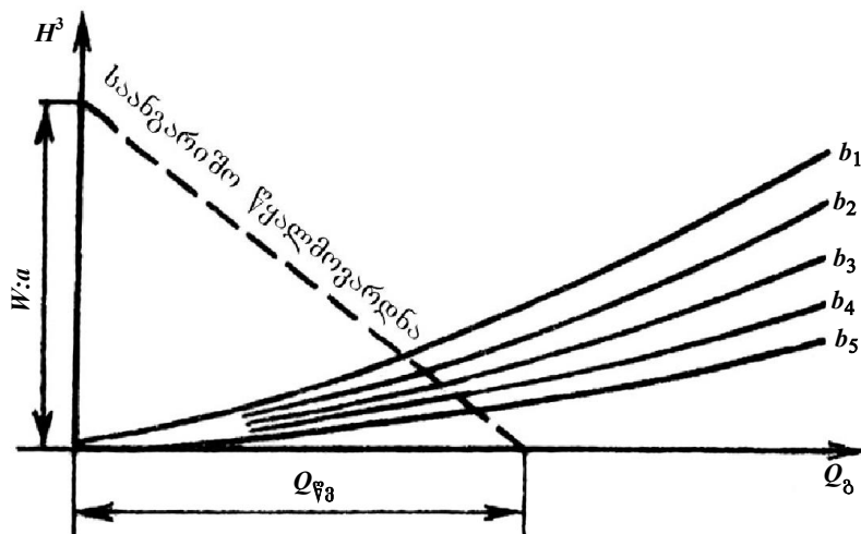
ნახ. 9.9. მიღების ხერტის საანგარიშო სქემა აკუმულაციის გათვალისწინებით
