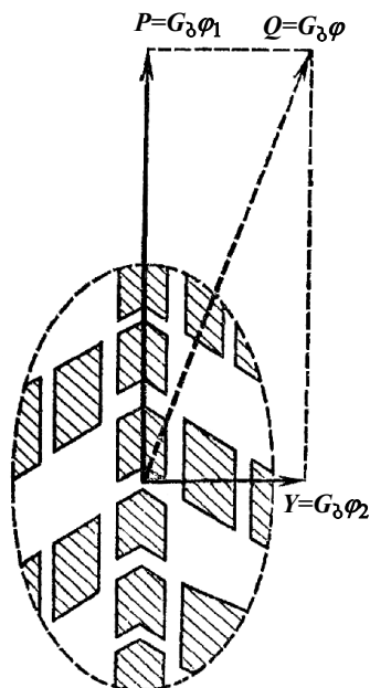
ნახ. 4.2. ავტომობილის ბორბალზედ მოქმედი გრძივი და განივი ძალების შეფარდება
