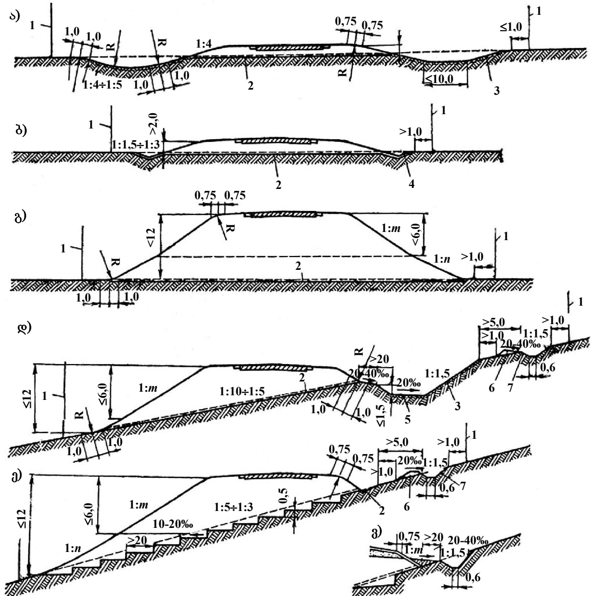
ნახ. 2.12. მიწის ვაკის განივი პროფილები ყრილებში:
