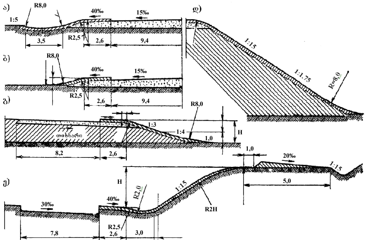
ნახ. 12.16. მიწის ვაკის მომრგვალებული განივი პროფილები.
