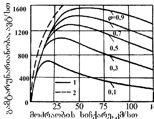
ნახ. 6.5. საავალი ზოლის თეორიული გამტარუნარიანობა ჩაჭიდების კოეფიციენტის სხვადასხვა მნიშვნელობისათვის: 1 – განტოლება 6.4-ის მიხედვით; 2 – განტოლება 6.5-ის მიხედვით
