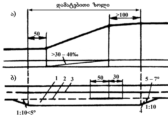
ნახ. 5.7. დამატებითი სავალი ზოლის სქემა აღმართზე:
