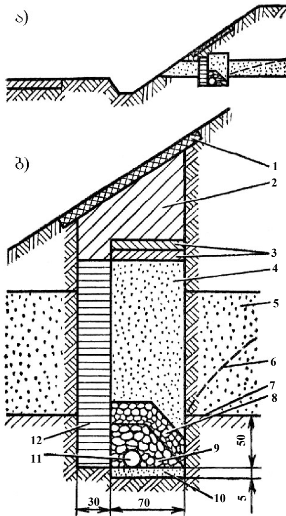
ნახ. 8.11. დამჭერი დრენაჟი:
