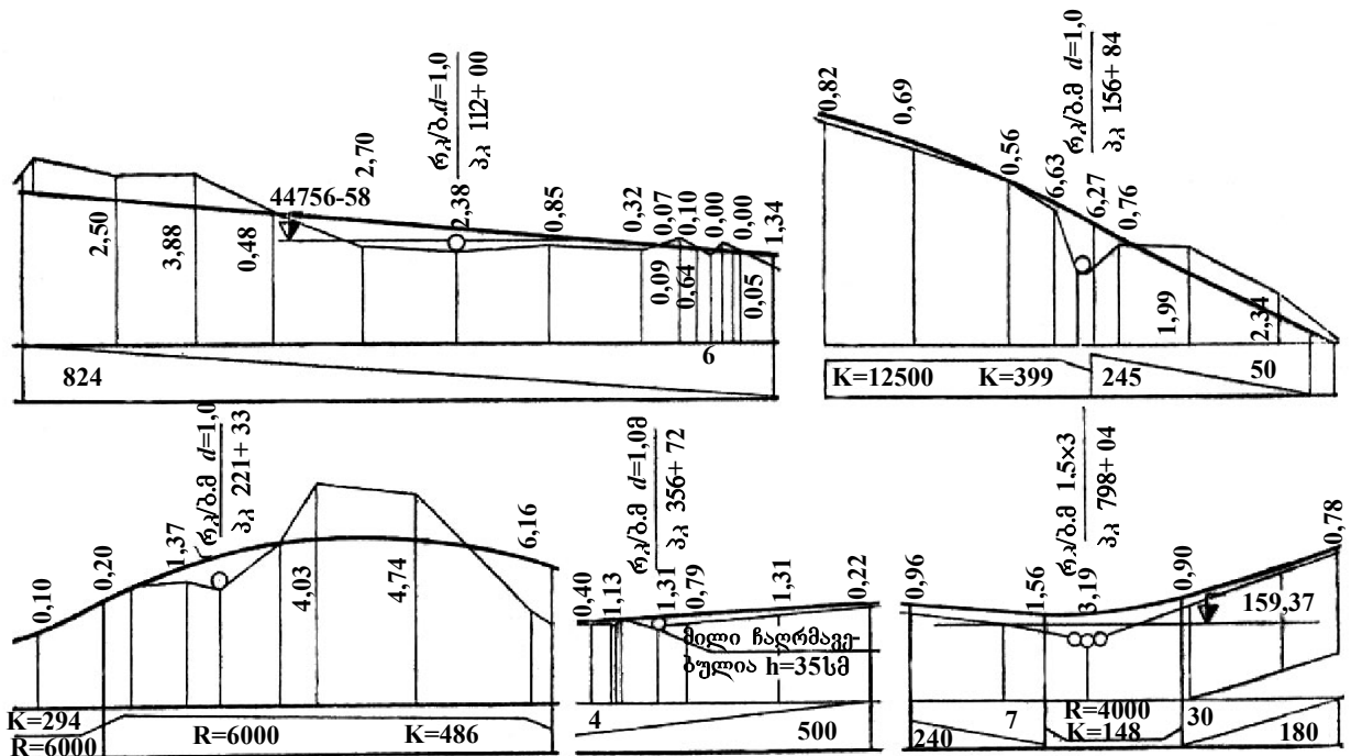
ნახ. 11.4. საპროექტო ხაზის დატანის მაგალითები წყალგადამშვებ მილებზე.
