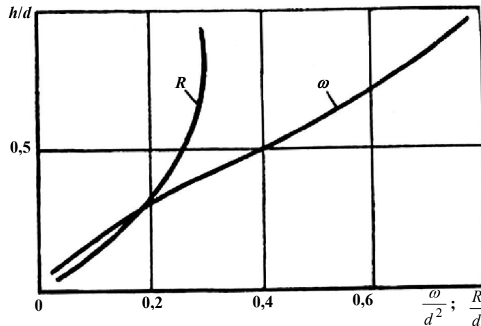
ნახ. 9.5. მრგვალი მილების საანგარიშო დამხმარე გრაფიკები
