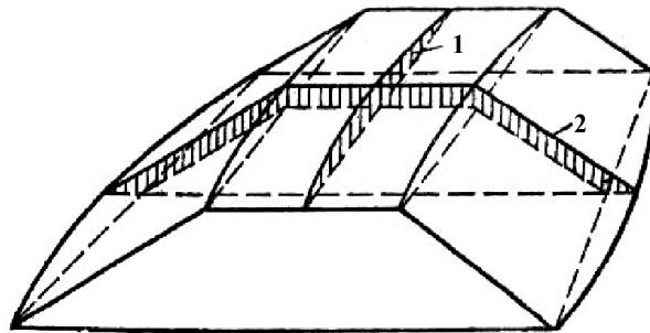
ნახ. 11.9. მიწის ვაკისის გაუთვალისწინებელი მოცულობა ვერტიკალური მრუდის მონაკვეთზე:
