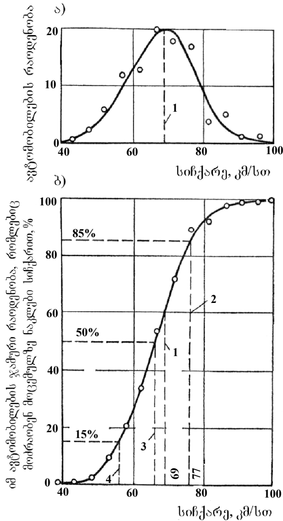
ნახ. 6.1. ავტომობილების სიჩქარეთა განაწილების კანონზომიერება ნაკადში მოძრაობისას:
