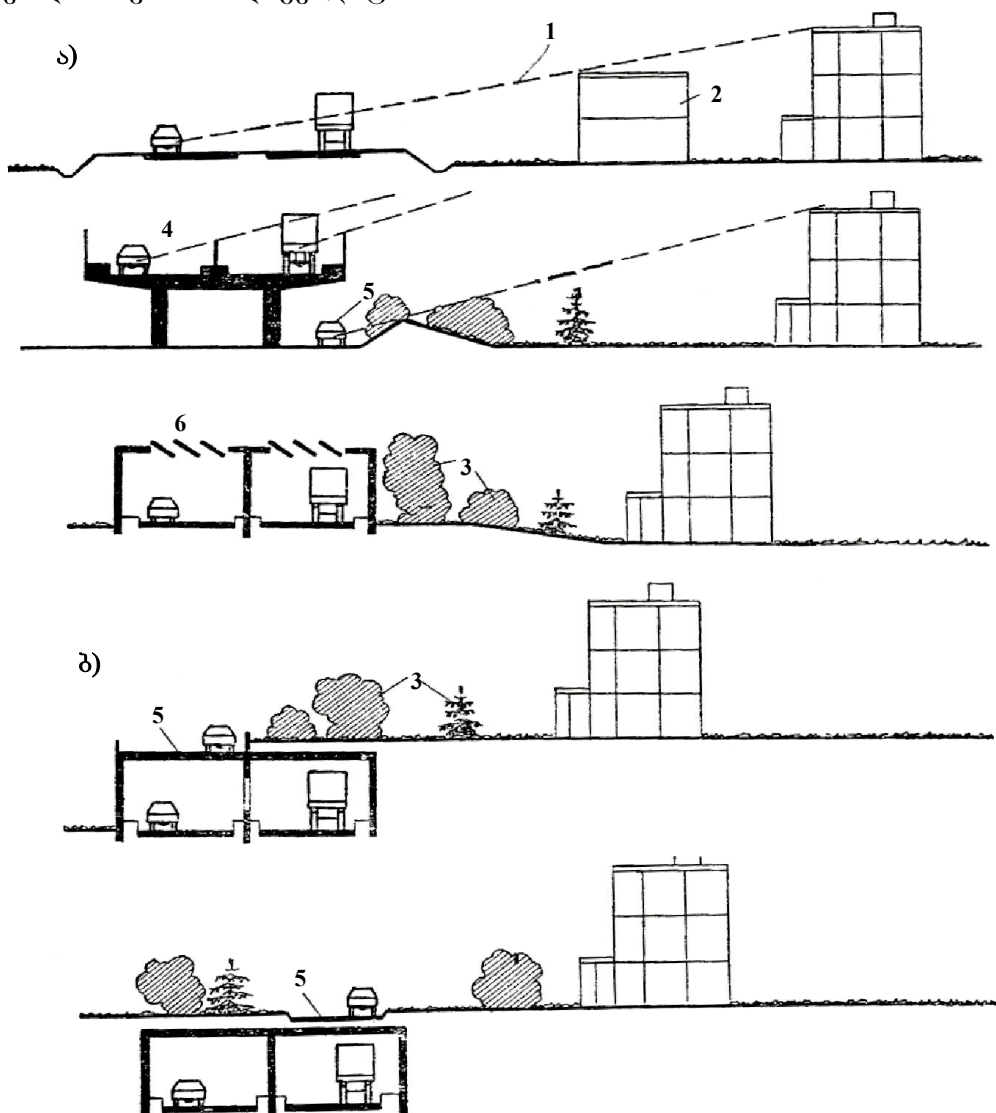
ნახ. 12.6. გზისპირა სივრცის დაცვა ხმაურისაგან:
