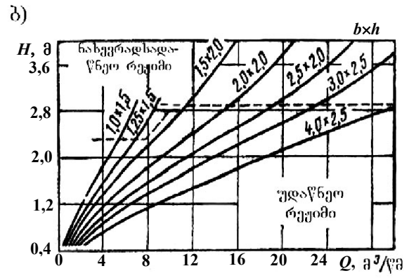
ნახ. 9.6. ტიპური უნიფიცირებული მილების გამტარუნარიანობის გრაფიკები: ა – მრგვალი მილებისათვის; ბ – სწორკუთხა მილებისათვის, ციფრები მრუდებზე - მილის ხერცები, მ
