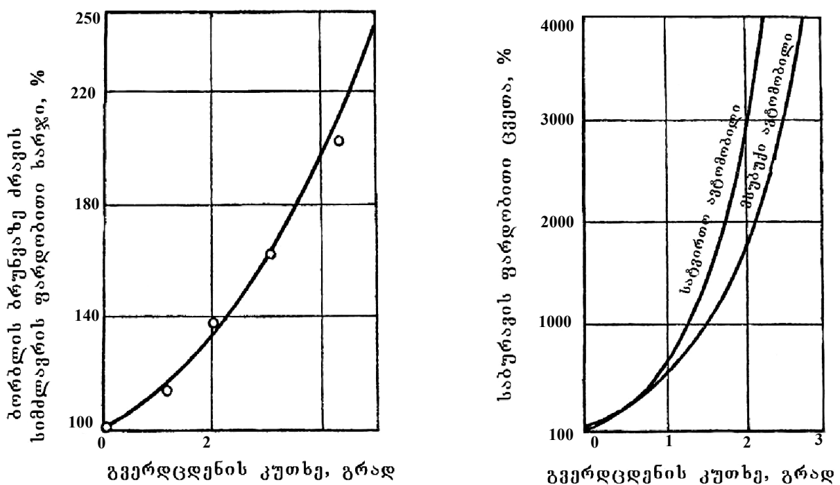
ნახ. 4.6. ავტომობილის მოძრაობის მახასიათებლები ბორბლის გვერდცდენით გორვის პირობებში a – სიმძლავრის დანახარჯები, b – საბურავის ცვეთა.
