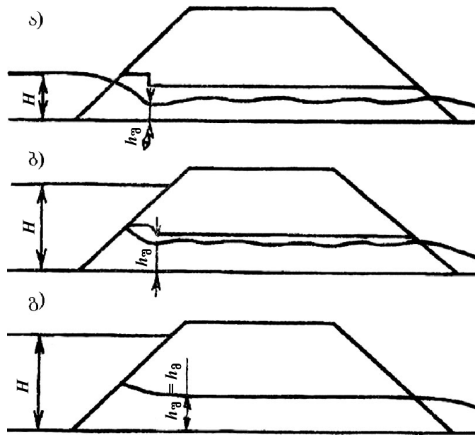
ნახ. 9.4. მიღების მუშაობის რეჟიმები: ა - უდაწნევო; ბ - ნახევრადდაწნევი; გ - დაწნევი
