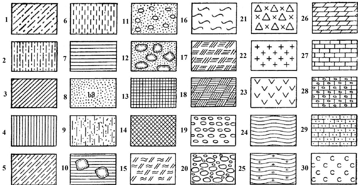
ნახ. 2.9. გრუნტებისა და მთის ქანების პირობითი აღნიშვნები საავტომობილო
