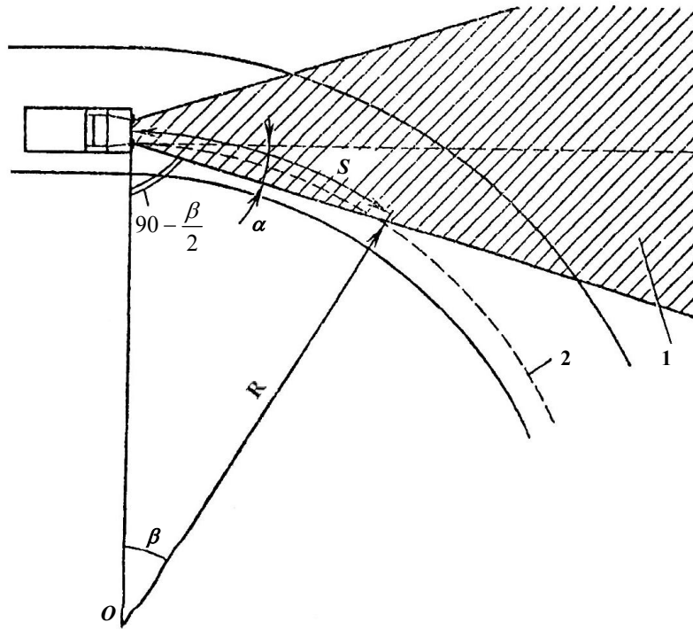
ნახ. 4.8. მრუდის რადიუსის განსაზღვრის სქემა ფარების შუქით განათების პირობიდან 1 - ფარებით განათებული ზონა; 2 - ავტომობილის ტრაექტორია
