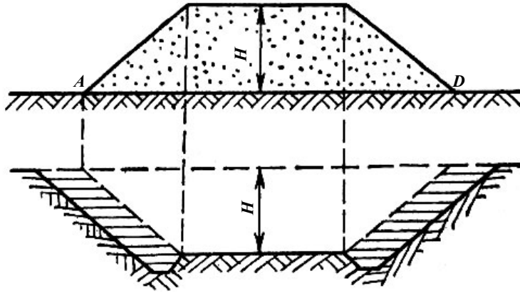
ნახ. 11.6. ტოლი მუშა ნიშნულების მქონე ყრილისა და ჭრილის მოცულობების განსაზღვრა
