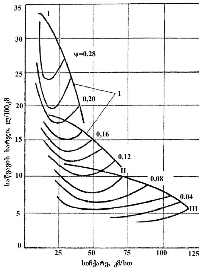
ნახ. 3.13. ეკონომიურ მახასიათებელთა გრაფიკის მაგალითი. ციფრები მრუდებზე ახასიათებენ საგზაო წინააღმდეგობათა სიდიდეს \varphi = f + i ; I-III მრუდეთა ჯგუფები I-III გადაცემებზე მოძრაობის შესაბამისი 1 – საწვავის მაქსიმალური ხარჯების მრუდები სხვადასხვა სიჩქარით მოძრაობისას.
