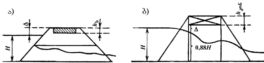
ნახ. 9.12. ყრილის სიმაღლის განსაზღვრის სქემა წყალგაღამშვებ ნაგებობასთან: ა – მილთან; ბ – მცირე ხილთან
