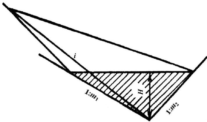
ნახ. 9.8. ტბორის მოცულობის დასადგენი სქემა
