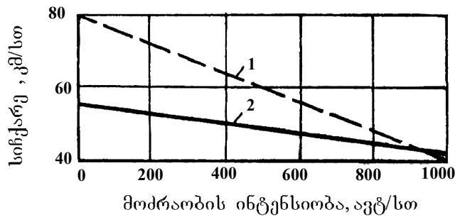
ნახ. 6.6. მოძრაობის საშუალო სიჩქარის დამოკიდებულება ნაკადის ინტენსიობისაგან: 1 – მხოლოდ მსუბუქი ავტომობილები; 2 – შერეული ნაკადი.
