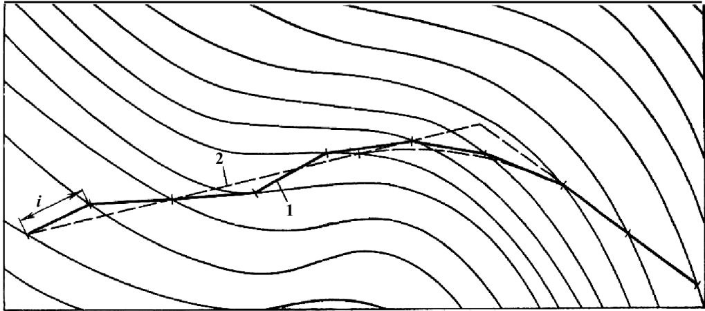
ნახ. 10.7. მოცემული ქანობით გზის ტრასირების ხერხები ჰორიზონტალებთან გეგმაზე: 1 – მოცემულია ქანობის ხაზი; 2 – ტრასა, მოცემულია ქანობის გამასწორებელი.
