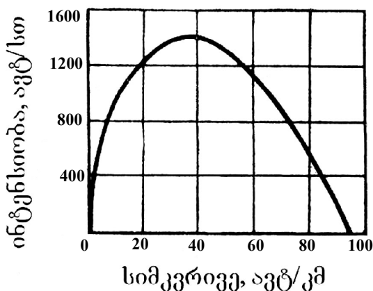
ნახ. 6.4. ავტომობილთა ნაკადის სიმკვრივისა და მოძრაობის ინტენსიობის დამოკიდებულების გრაფიკი
