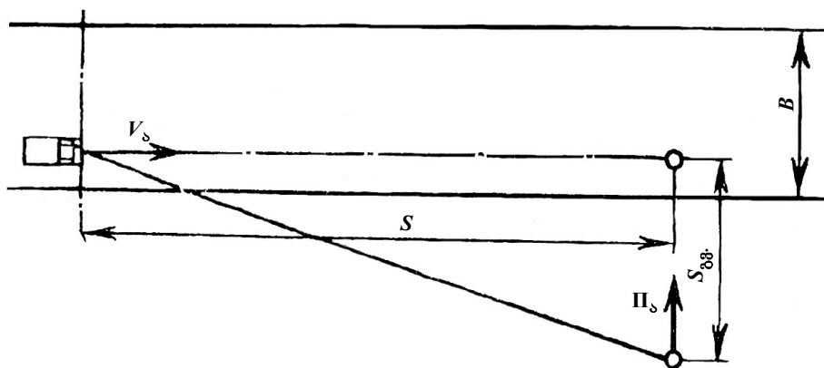
ნახ. 4.18. გვერდითი მხედველობის მანძილის საანგარიშო სქემა B – სავალი ნაწილის სიგანე
