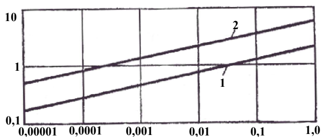
ნახ. 9.3. ნაკადის ჩამოღინების სიჩქარის დამოკიდებულება აუზის ქანობზე:
