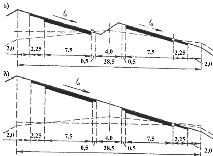
ნახ. 4.16. ვირაუის განივი პროფილები ავტომაგისტრალებზე
