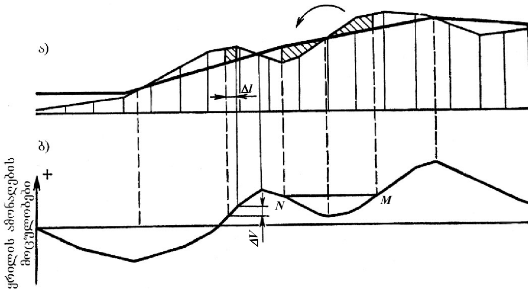
ნახ. 11.10. მიწის მასების განაწილების გრაფიკის შედგენა: 1 – გრძივი პროფილი; 2 – მიწის მასების განაწილების გრაფიკი.
