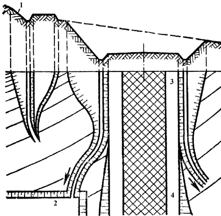
ნახ. 8.5. სამთო არხებიდან და კიუვეტებიდან წყლის გადაშვება რეზერვებში: 1 – სამთო არხი; 2 – რეზერვი; 3 – ჭრილი; 4 – ყრილი.
