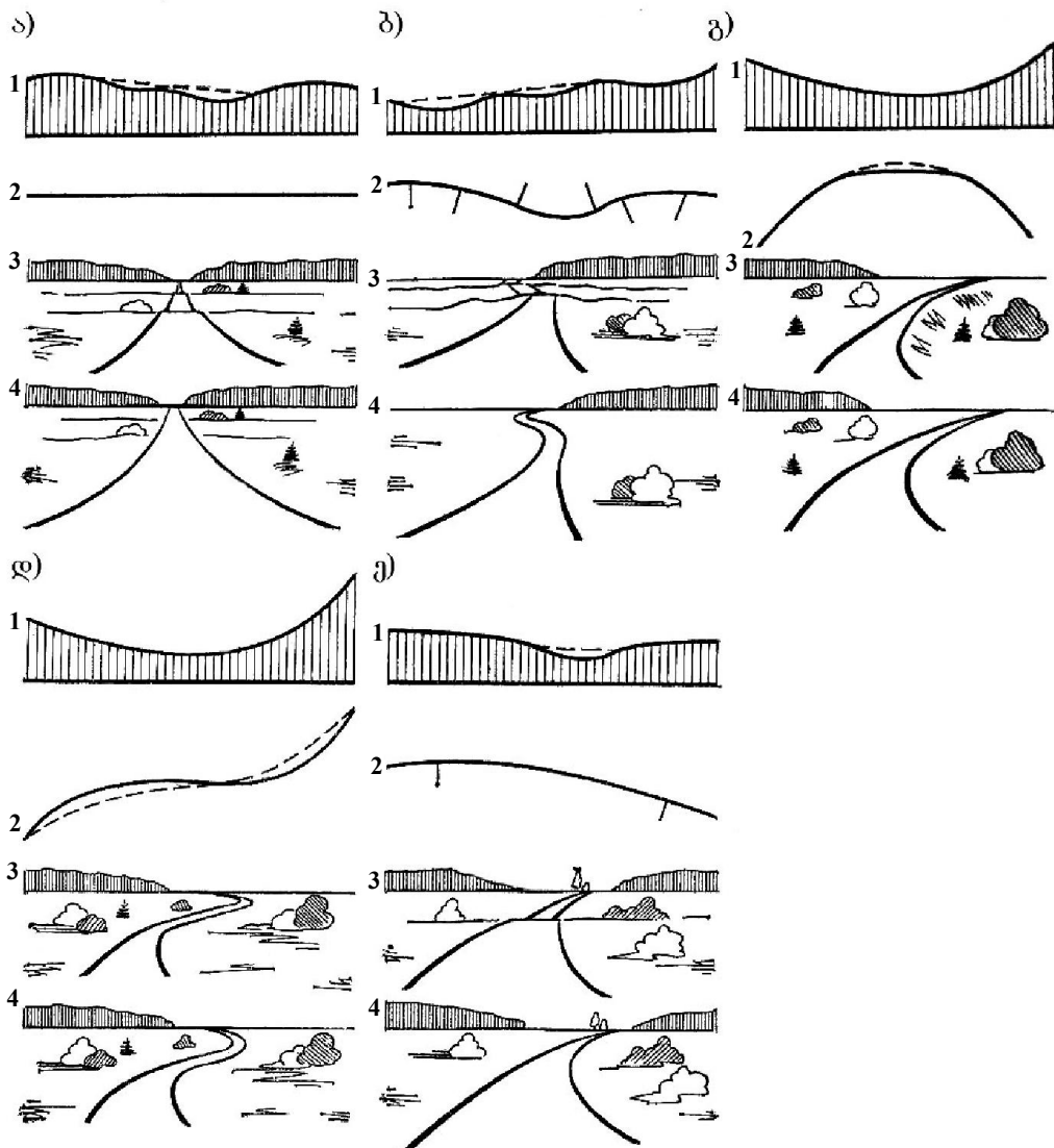
ნახ. 12.9. ტრასის ელემენტების არახელსაყრელი შესამება, რის შედეგადაც მძღოლისათვის გაურკვეველია გზის შემდგომი მიმართულება:
