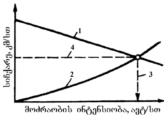
ნახ. 6.7. გზის გამტარუნარიანობის დამოკიდებულება მოძრაობის სიჩქარისაგან: 1 – ნაკადის სიჩქარის დამოკიდებულება ინტენსიობისაგან; 2 – გამტარუნარიანობა გათვლილი ავტომობილებს შორის ინტერვალებით; 3 – სავალი ზოლის გამტარუნარიანობა ტიპურ პირობებში; 4 – სიჩქარე ტიპური გამტარუნარიანობისას
