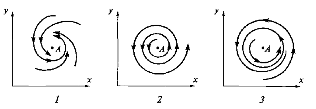
Рис.2. Три различных случая структурно устойчивого поведения взаимодействующей системы добра и зла в сознании индивида
