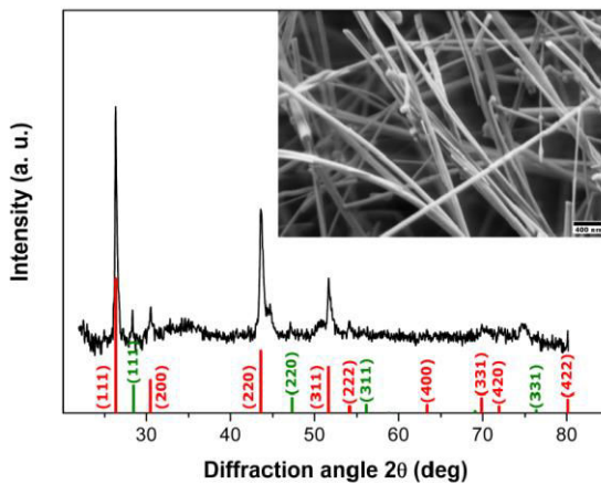
ნახ.7. 350°C ტემპერატურაზე მიღებული InP+Ga გული-გარსი ტიპის ნანომავთულების რენტგენოფაზური ანალიზი და (რემ) სურათი. (წითელი ფერით აღნიშნულია არაორგანული კრისტალური სტრუქტურის ორიენტაციები ICSD73-1983; მწვანე ფერი ეკუთვნის Si-ის ფუძემშრეს)
